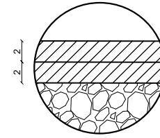
PAVIMENTAÇÃO 4cm
