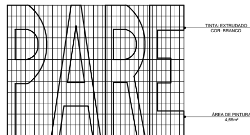
PINTURA VIÁRIA DE PARADA OBRIGATÓRIA SEM ESCALA
