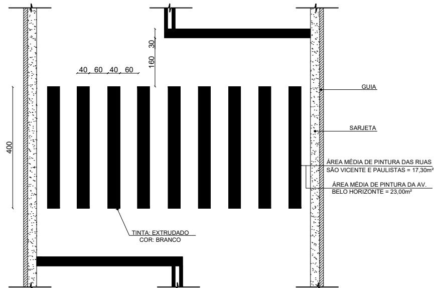
FAIXA DE PEDESTRE ZEBRADA SEM ESCALA
