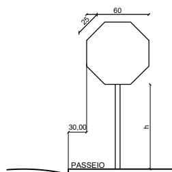
PLACA - PARADA OBRIGATÓRIA (R-1) SEM ESCALA
