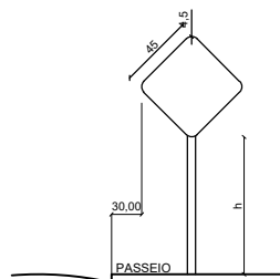
PLACA - PASSAGEM SINALIZADA DE PEDESTRES (A-32b) SEM ESCALA
