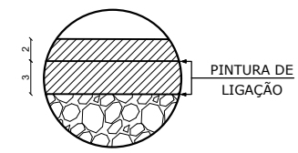
PAVIMENTAÇÃO 5cm
