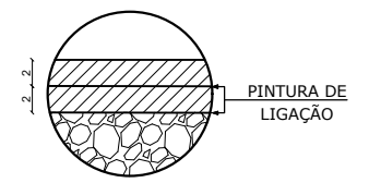
PAVIMENTAÇÃO 4cm
