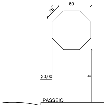
PLACA - PARADA OBRIGATÓRIA (R-1) SEM ESCALA
