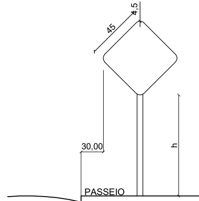
PLACA - LOMBADA (A-18) SEM ESCALA
