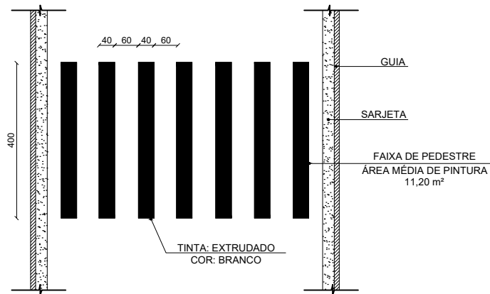
FAIXA DE PEDESTRE ZEBRADA SEM ESCALA
