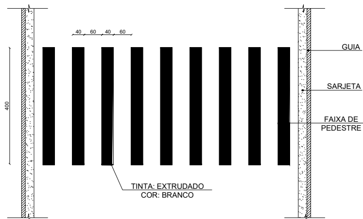
FAIXA DE PEDESTRE ZEBRADA SEM ESCALA
