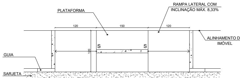
REBAIXAMENTO DE CALÇADA TIPO D - NBR 9050 SEM ESCALA
