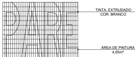
PINTURA VIÁRIA DE PARADA OBRIGATÓRIA SEM ESCALA
