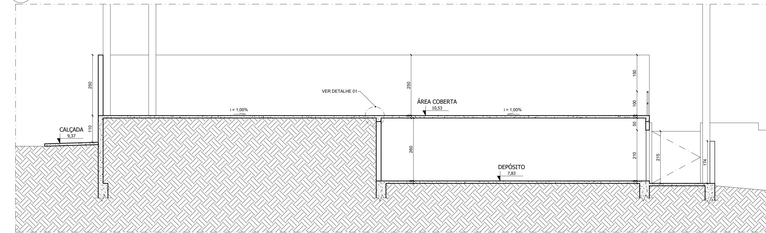
13 CORTE CC ESCALA 1:75
