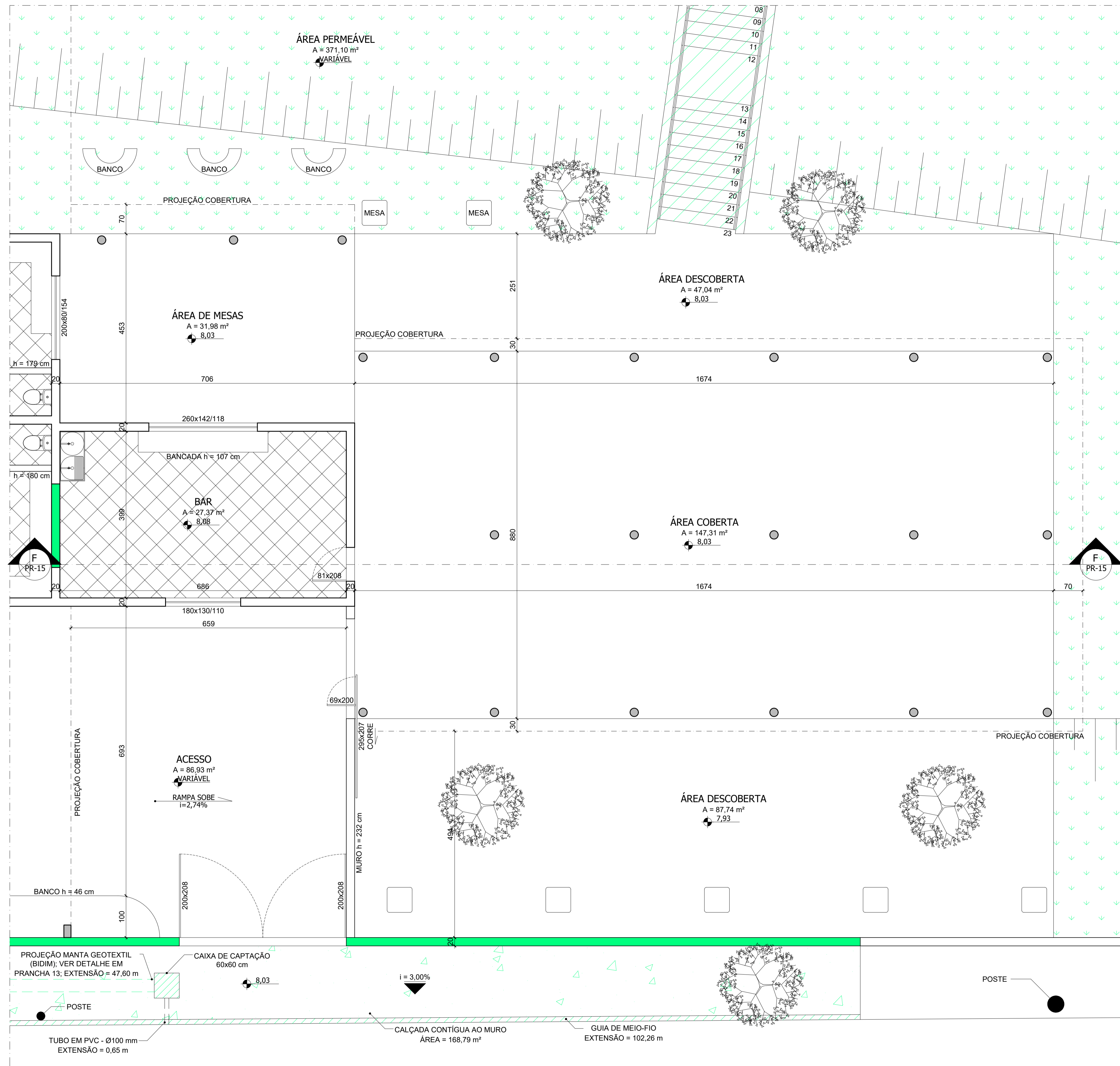
09 PLANTA - BAR (ACRÉSCIMO) ESCALA 1:50
