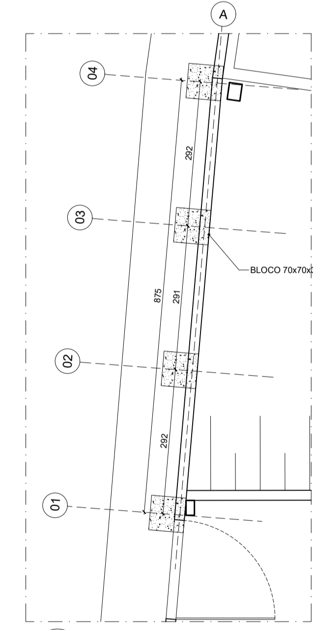
31 PLANTA ESTACAS - TRECHO 05 ESCALA 1:75
