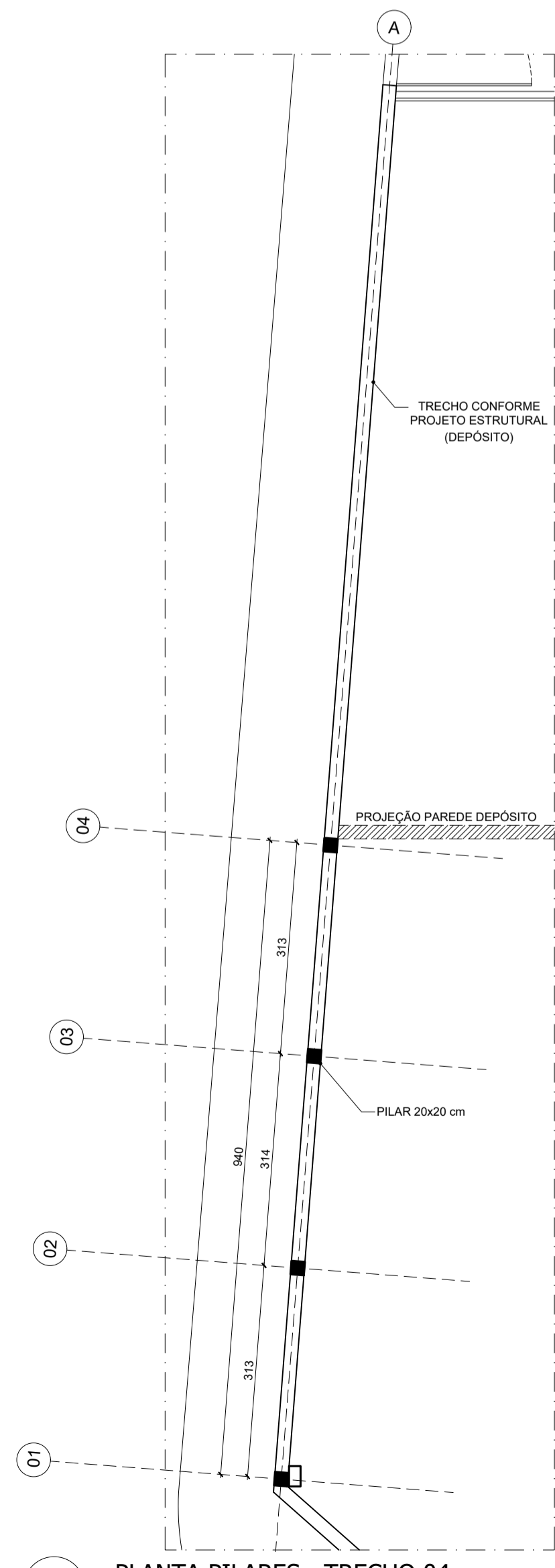
28 PLANTA PILARES - TRECHO 04 ESCALA 1:75
