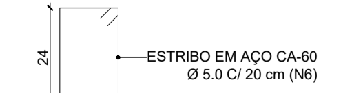
37 DET. VIGA INFERIOR / INTERMEDIÁRIA 01 ESCALA 1:5
