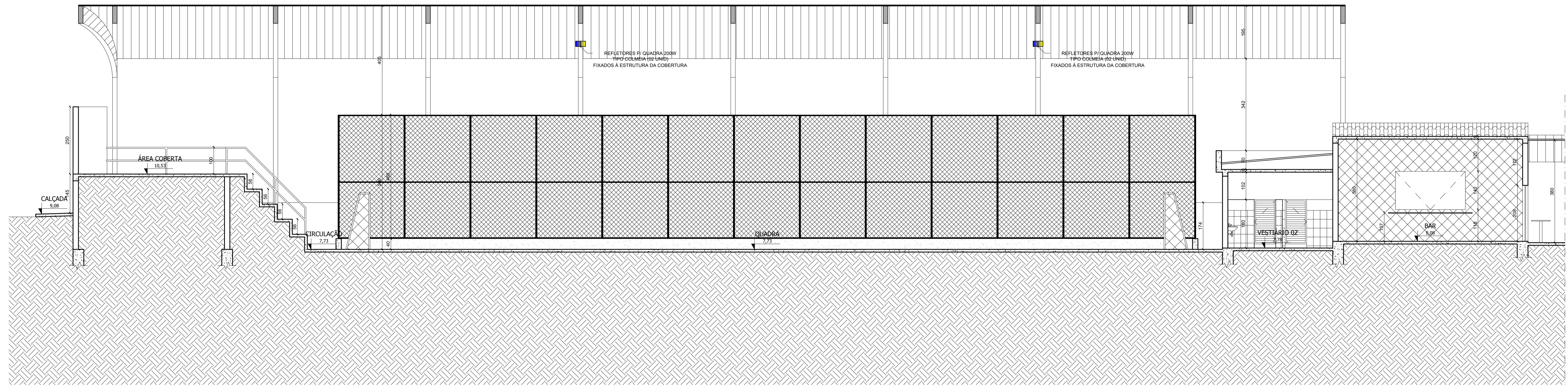
44 CORTE FF ESCALA 1:75
