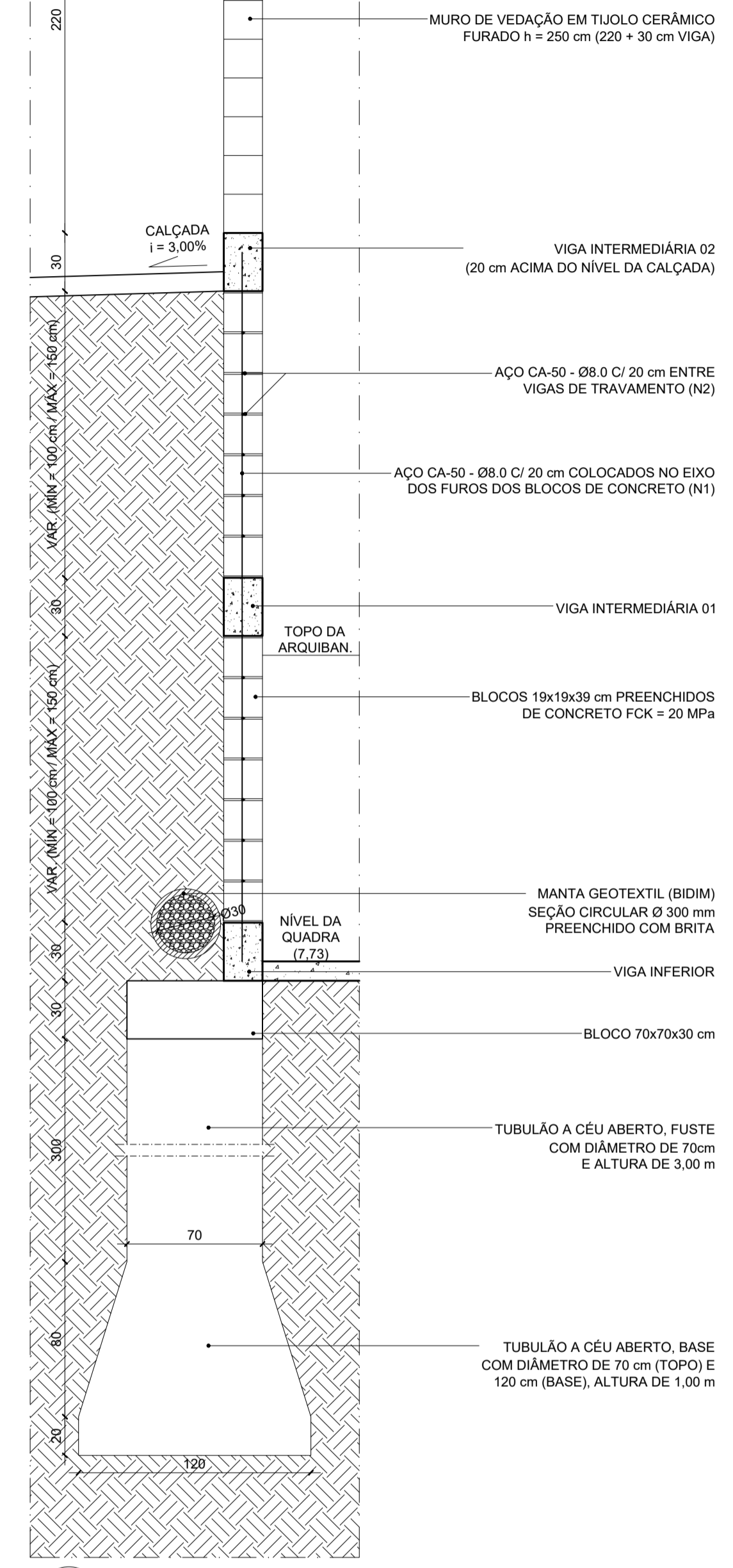
33 SEÇÃO TRANSVERSAL - TRECHOS 02/03 ESCALA 1:25
