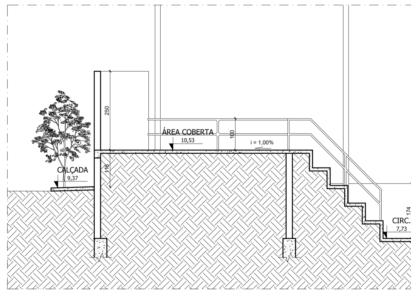
12 CORTE BB ESCALA 1:75
