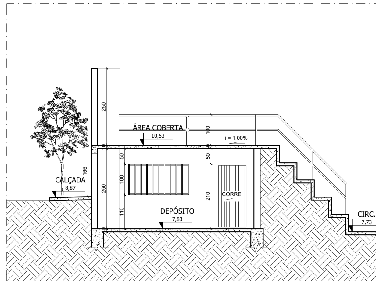
11 CORTE AA ESCALA 1:75
