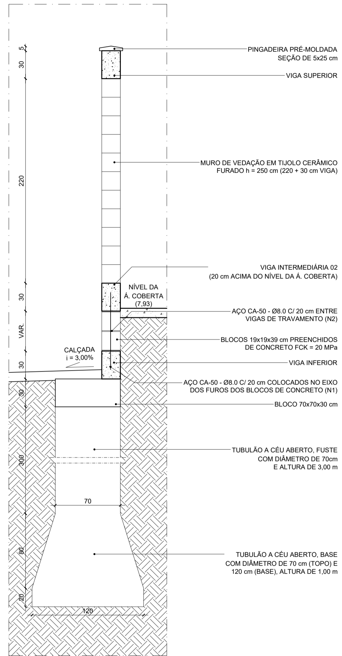
32 SEÇÃO TRANSVERSAL - TRECHO 01 ESCALA 1:25
