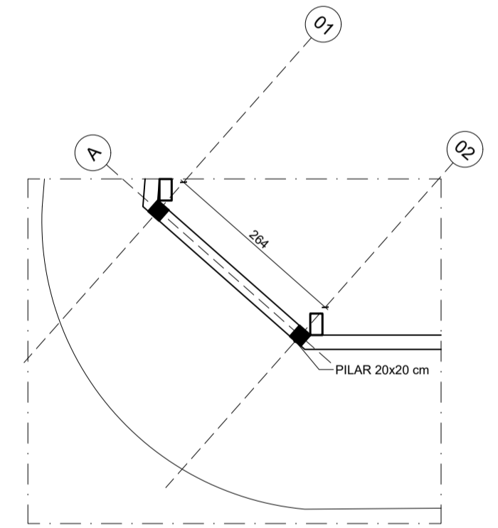
26 PLANTA PILARES - TRECHO 03 ESCALA 1:75
