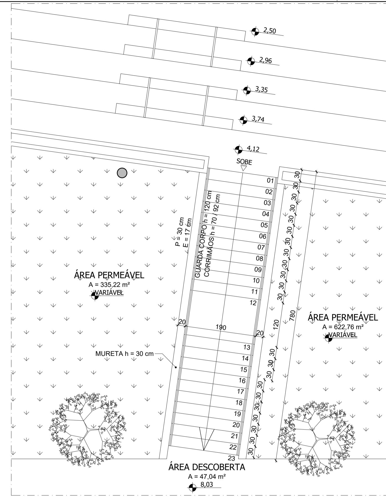
14 PLANTA - ESCADA ESCALA 1:50
