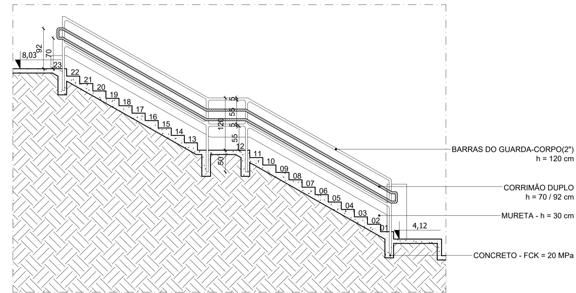
15 SEÇÃO LONGITUDINAL - ESCADA ESCALA 1:50
