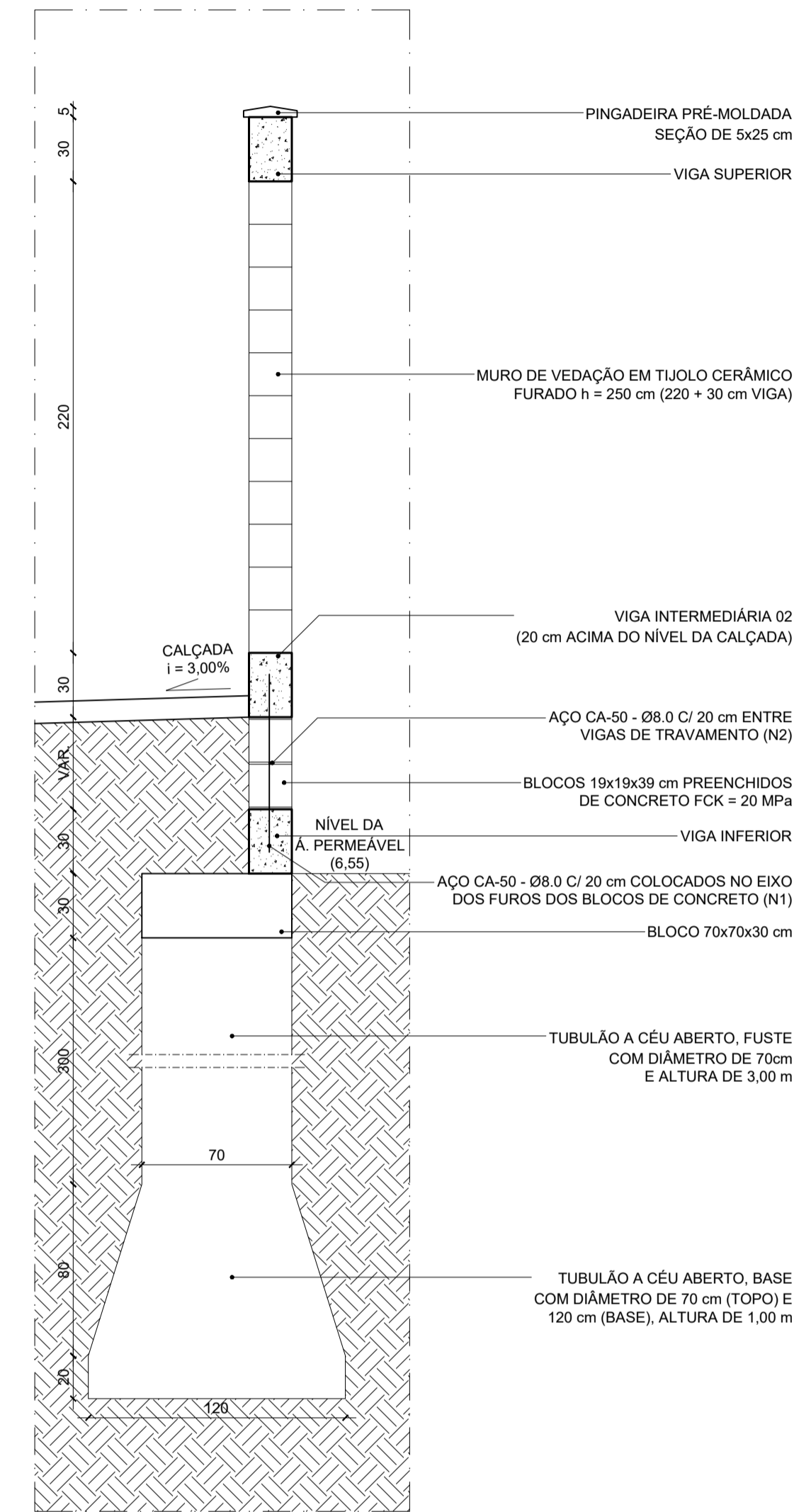
35 SEÇÃO TRANSVERSAL - TRECHO 05 ESCALA 1:25
