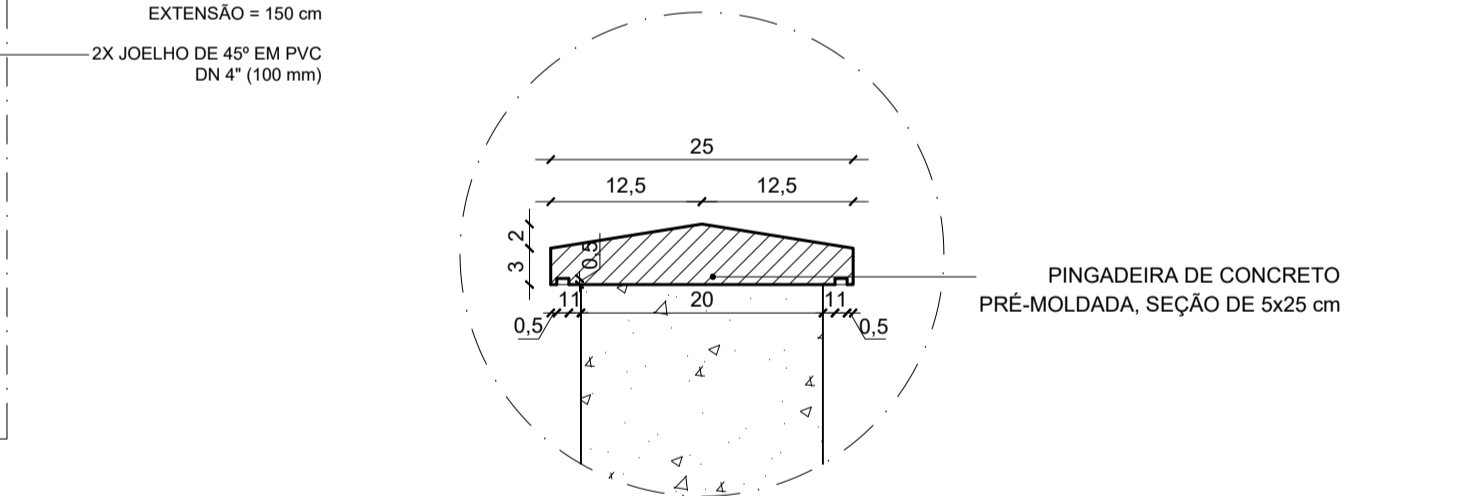
21 DETALHE PINGADEIRA ESCALA 1:5
