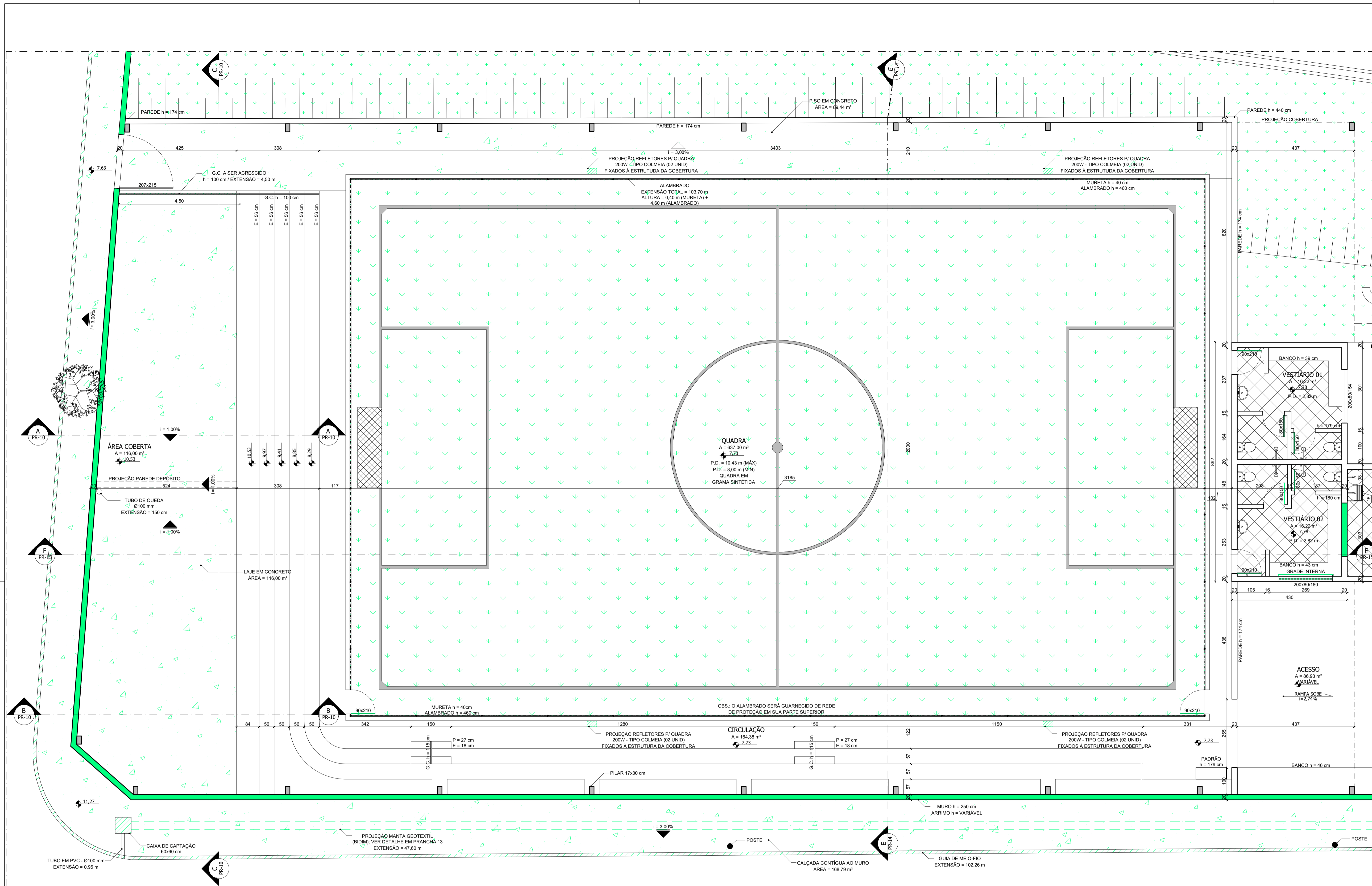
08 PLANTA - QUADRA (ACRÉSCIMO) ESCALA 1:75
