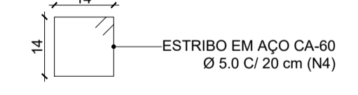
36 DETALHE PILARES ESCALA 1:10
