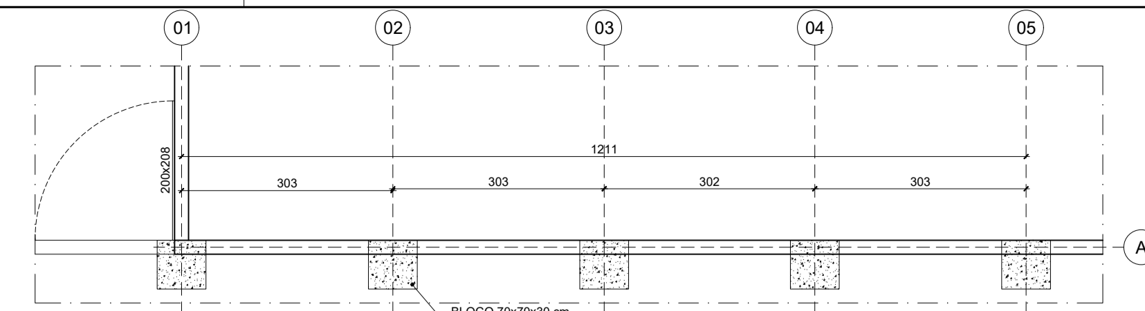
23 PLANTA ESTACAS - TRECHO 01 ESCALA 1:75
