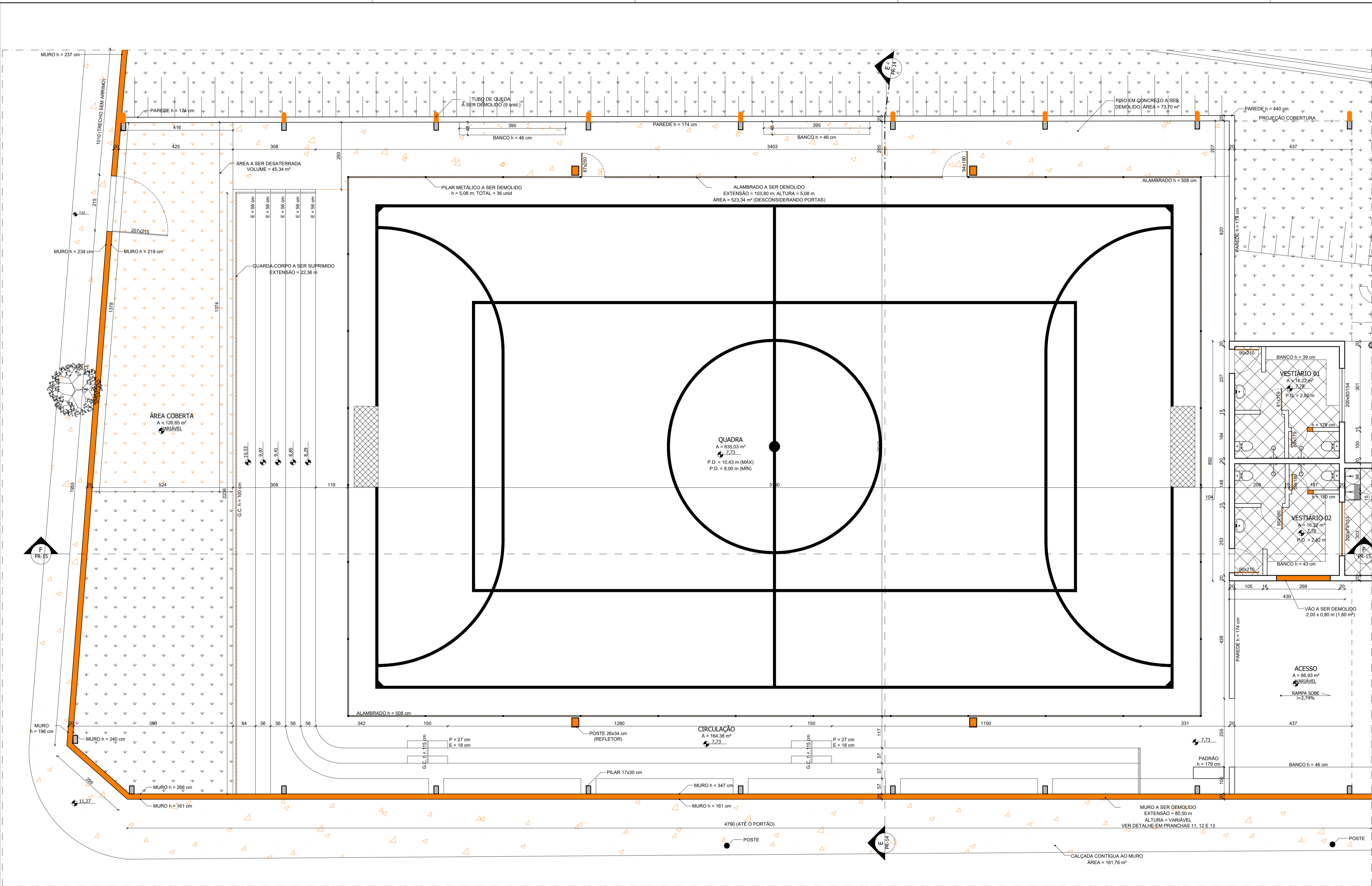
06 PLANTA - QUADRA (DEMOLIÇÃO) ESCALA 1:75
