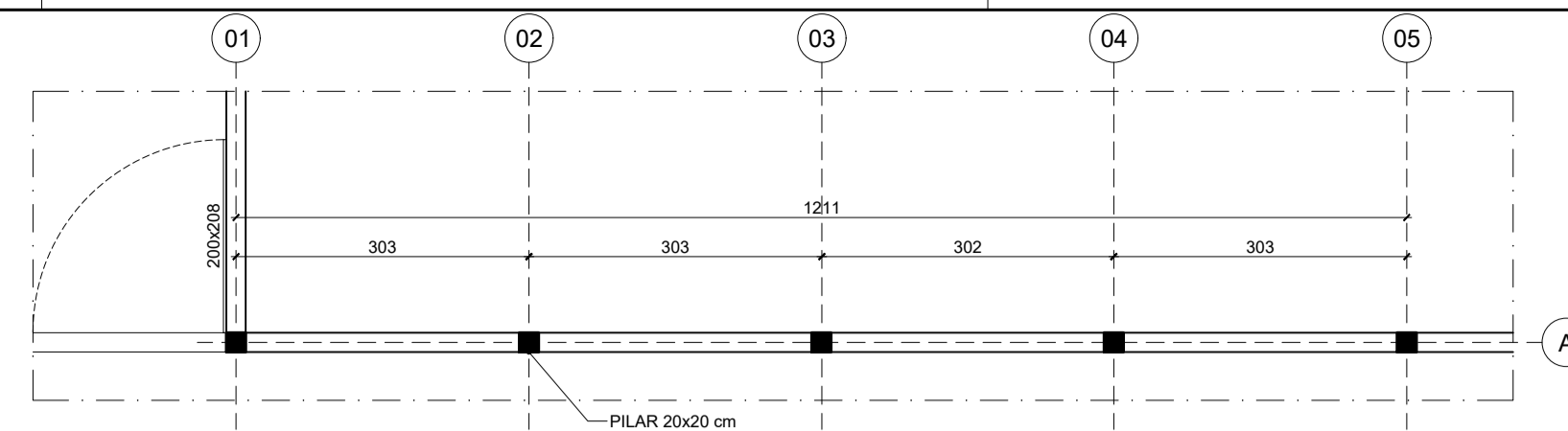
22 PLANTA PILARES - TRECHO 01 ESCALA 1:75
