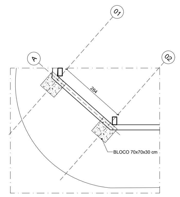
27 PLANTA ESTACAS - TRECHO 03 ESCALA 1:75
