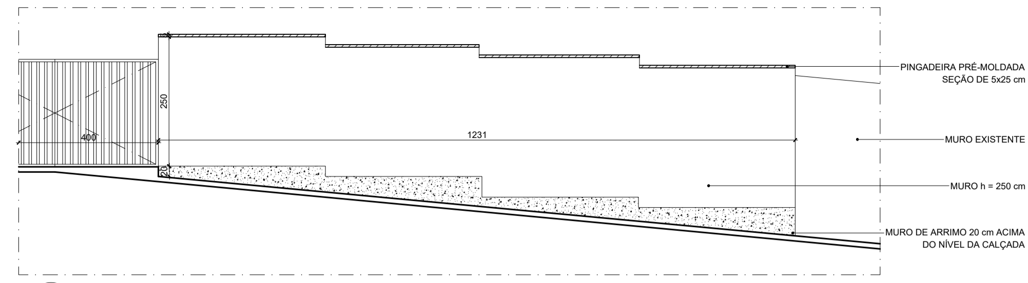
17 ELEVÇÃO 01 ESCALA 1:75
