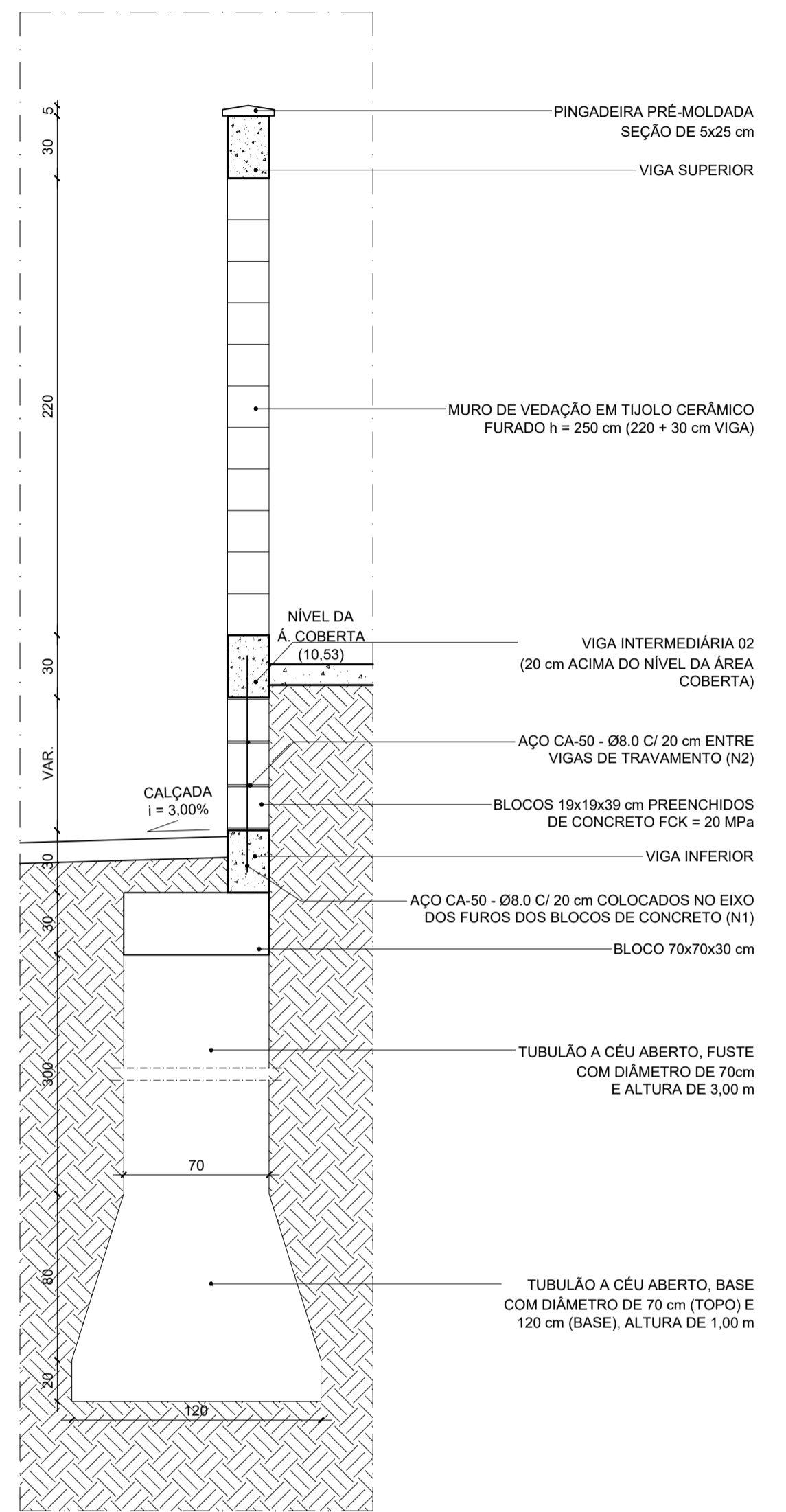
34 SEÇÃO TRANSVERSAL - TRECHO 04 ESCALA 1:25
