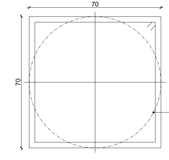
33 SEÇÃO TRANSVERSAL - TRECHOS 02/03 ESCALA 1:25
