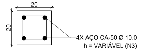
36 DETALHE PILARES ESCALA 1:10
