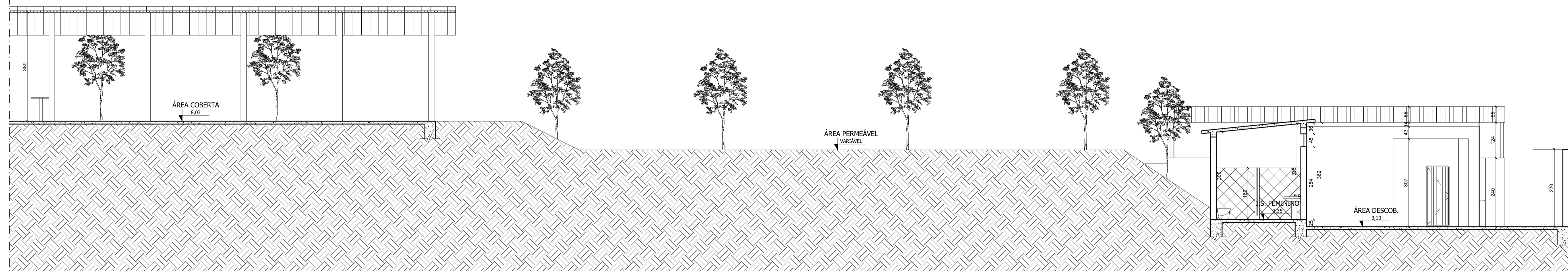
45 CORTE FF (CONTINUAÇÃO) ESCALA 1:75
