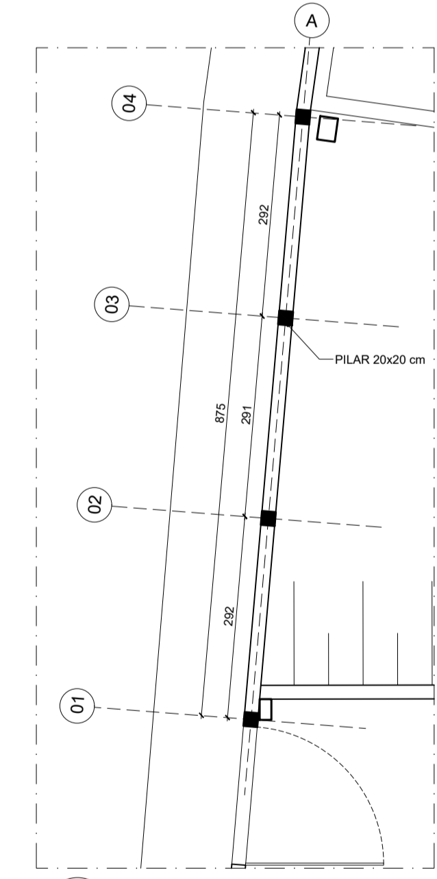
30 PLANTA PILARES - TRECHO 05 ESCALA 1:75
