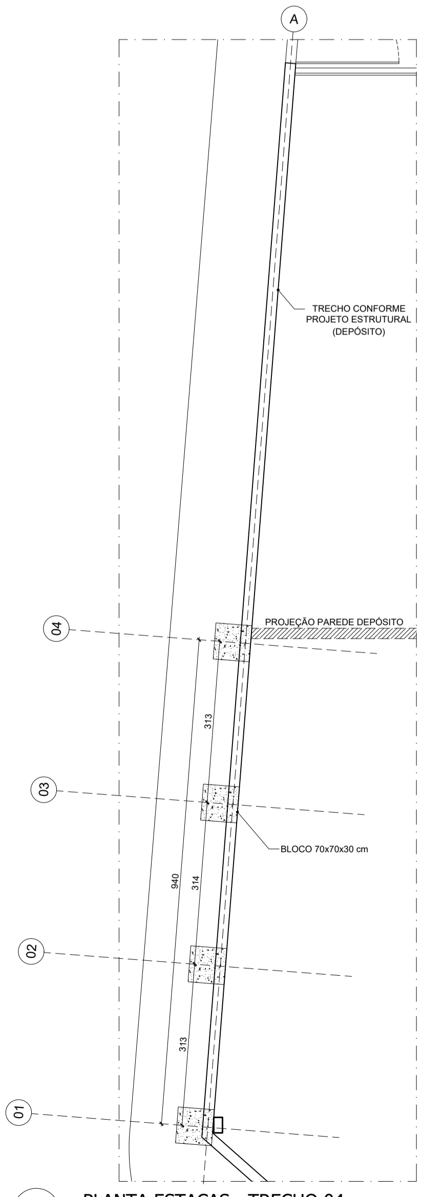
29 PLANTA ESTACAS - TRECHO 04 ESCALA 1:75
