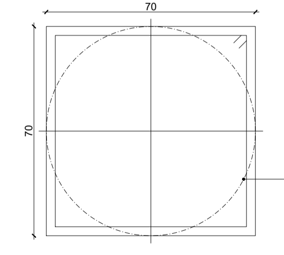
35 SEÇÃO TRANSVERSAL - TRECHOS 02/03 ESCALA 1:25
