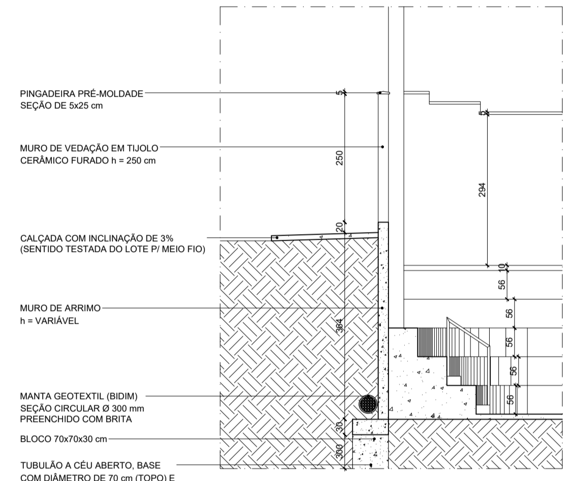
22 CORTE DD ESCALA 1:75
