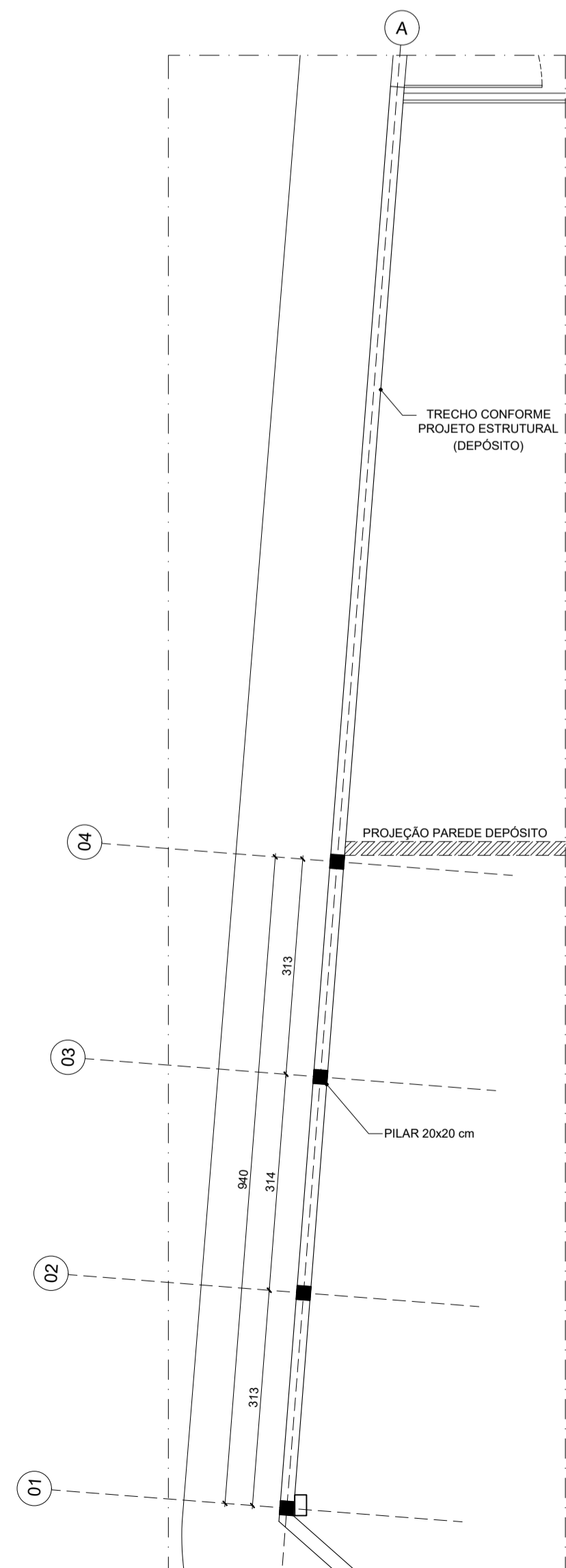
30 PLANTA PILARES - TRECHO 04 ESCALA 1:75
