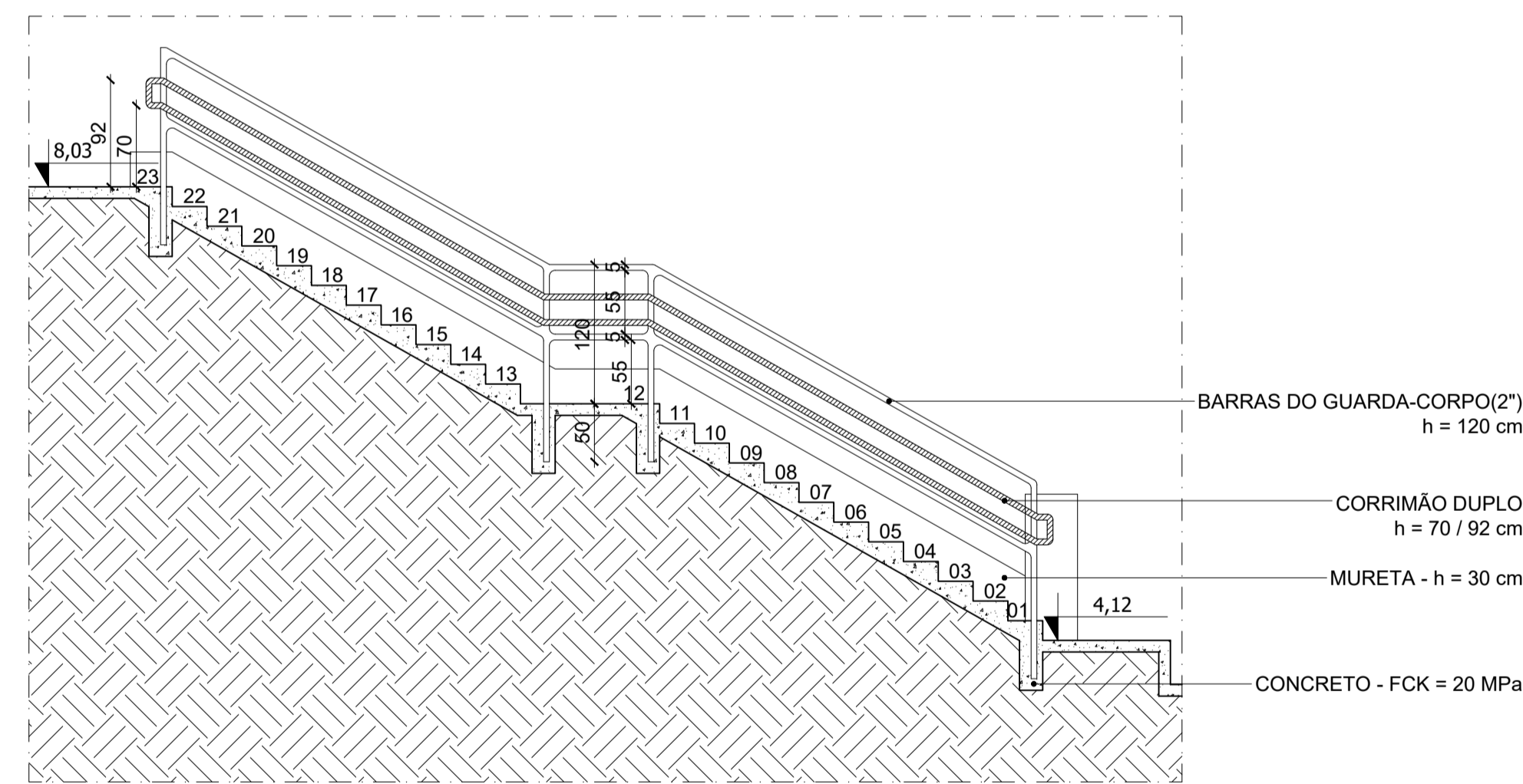
17 SEÇÃO LONGITUDINAL - ESCADA ESCALA 1:50
