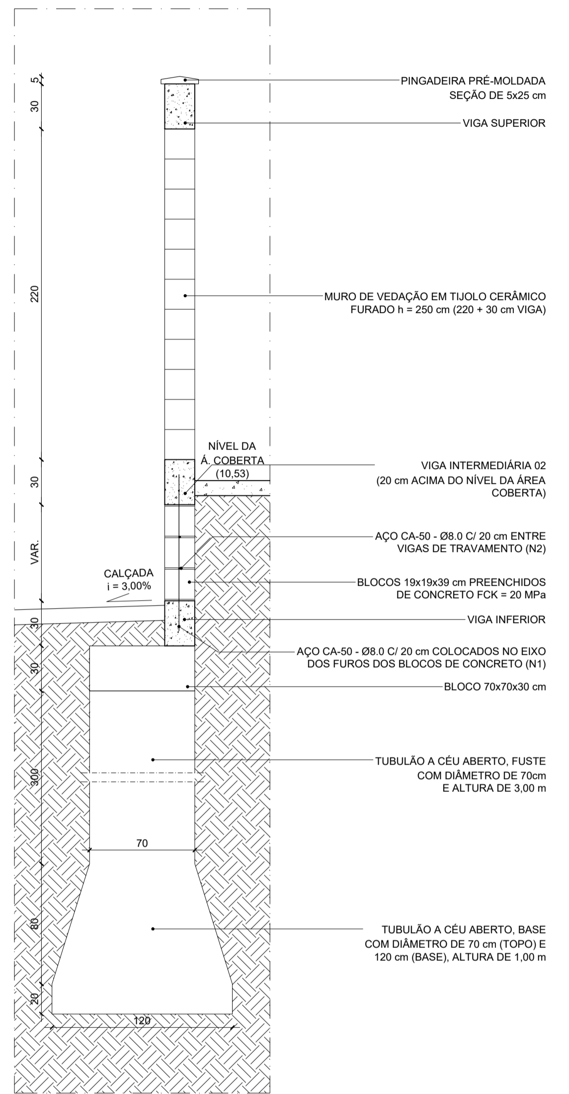
36 SEÇÃO TRANSVERSAL - TRECHO 04 ESCALA 1:25
