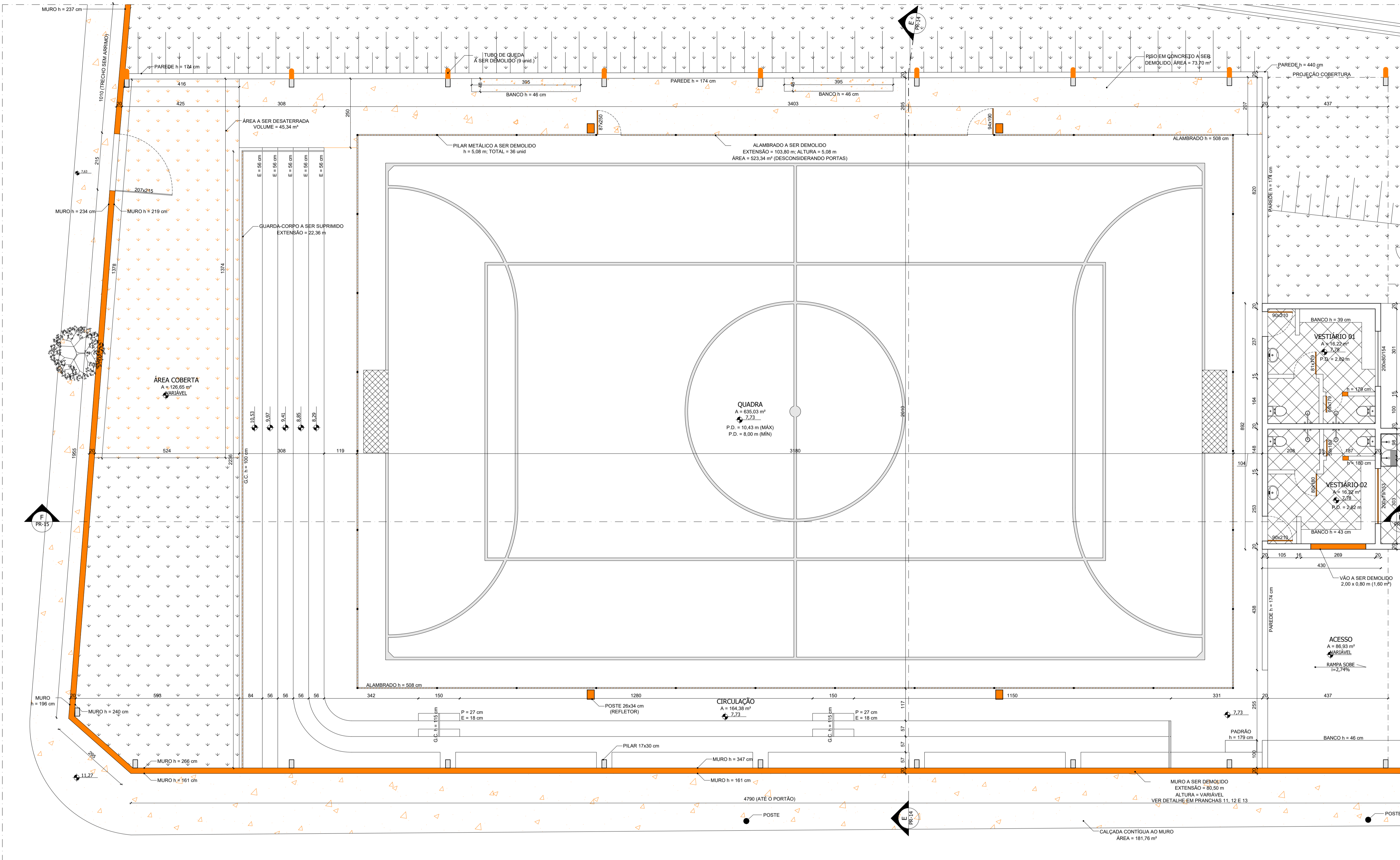
06 PLANTA - QUADRA (DEMOLIÇÃO)
