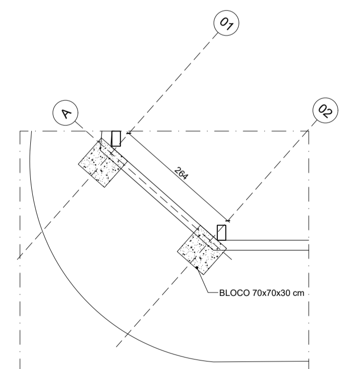
29 PLANTA ESTACAS - TRECHO 03 ESCALA 1:75
