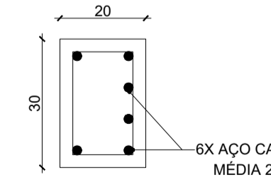
40 DET. VIGA INTERMEDIÁRIA 02 / SUPERIOR ESCALA 1:5
