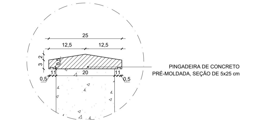
23 DETALHE PINGADEIRA ESCALA 1:5
