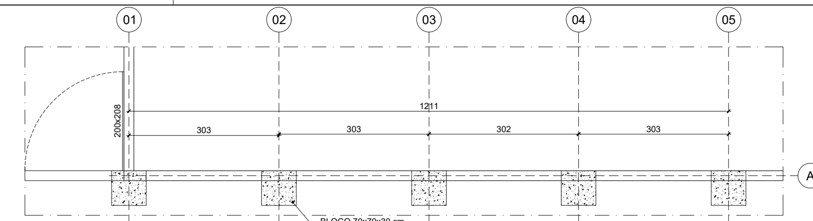
25 PLANTA ESTACAS - TRECHO 01 ESCALA 1:75
