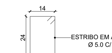
40 DET. VIGA INTERMEDIÁRIA 02 / SUPERIOR ESCALA 1:5
