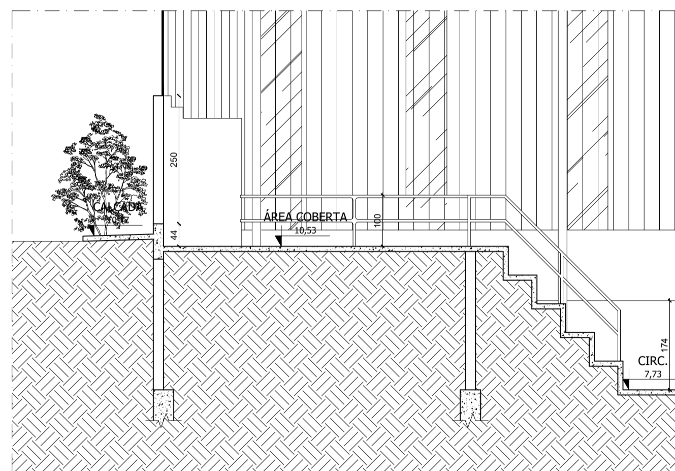
14 CORTE BB ESCALA 1:75
