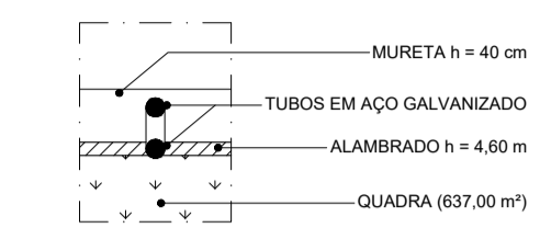
09 DETALHE - REFORÇO ALAMBRADO ESCALA 1:25
