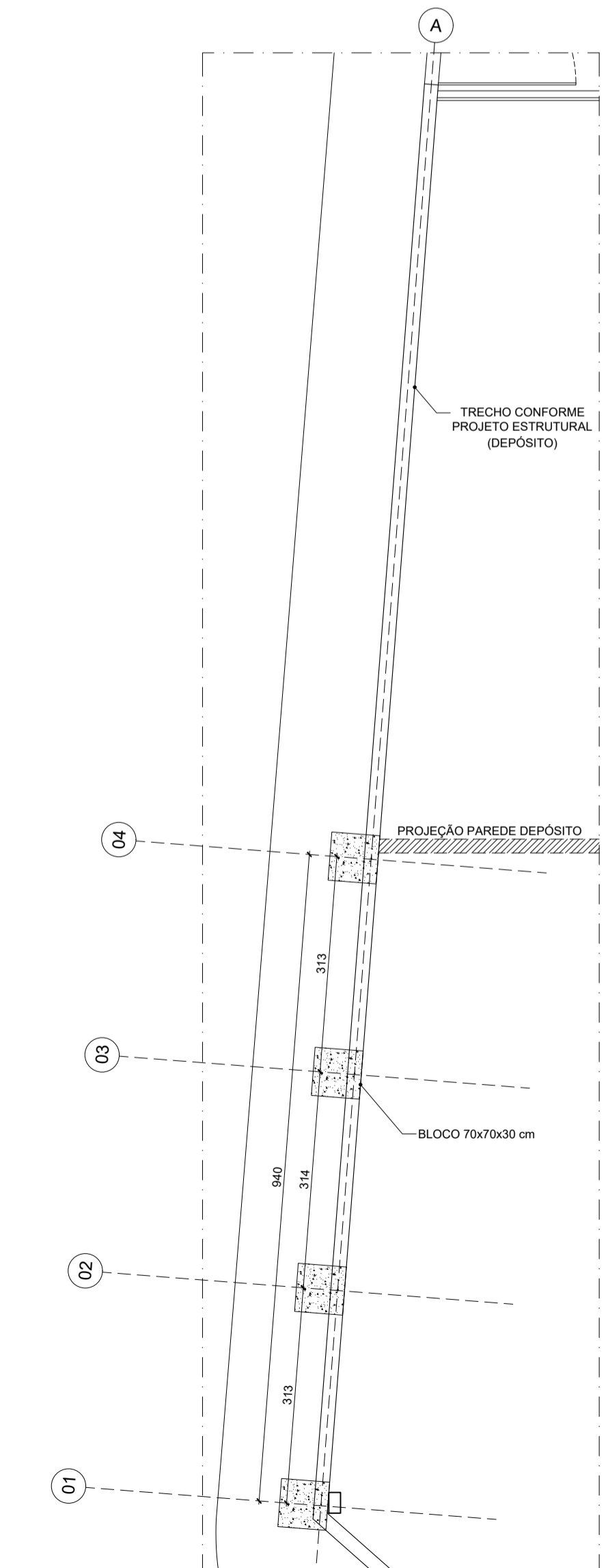
31 PLANTA ESTACAS - TRECHO 04 ESCALA 1:75
