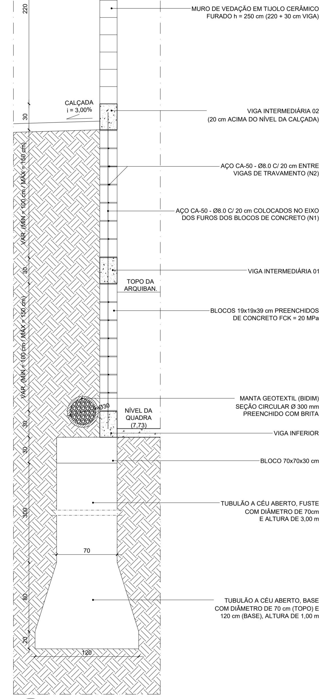
35 SEÇÃO TRANSVERSAL - TRECHOS 02/03 ESCALA 1:25
