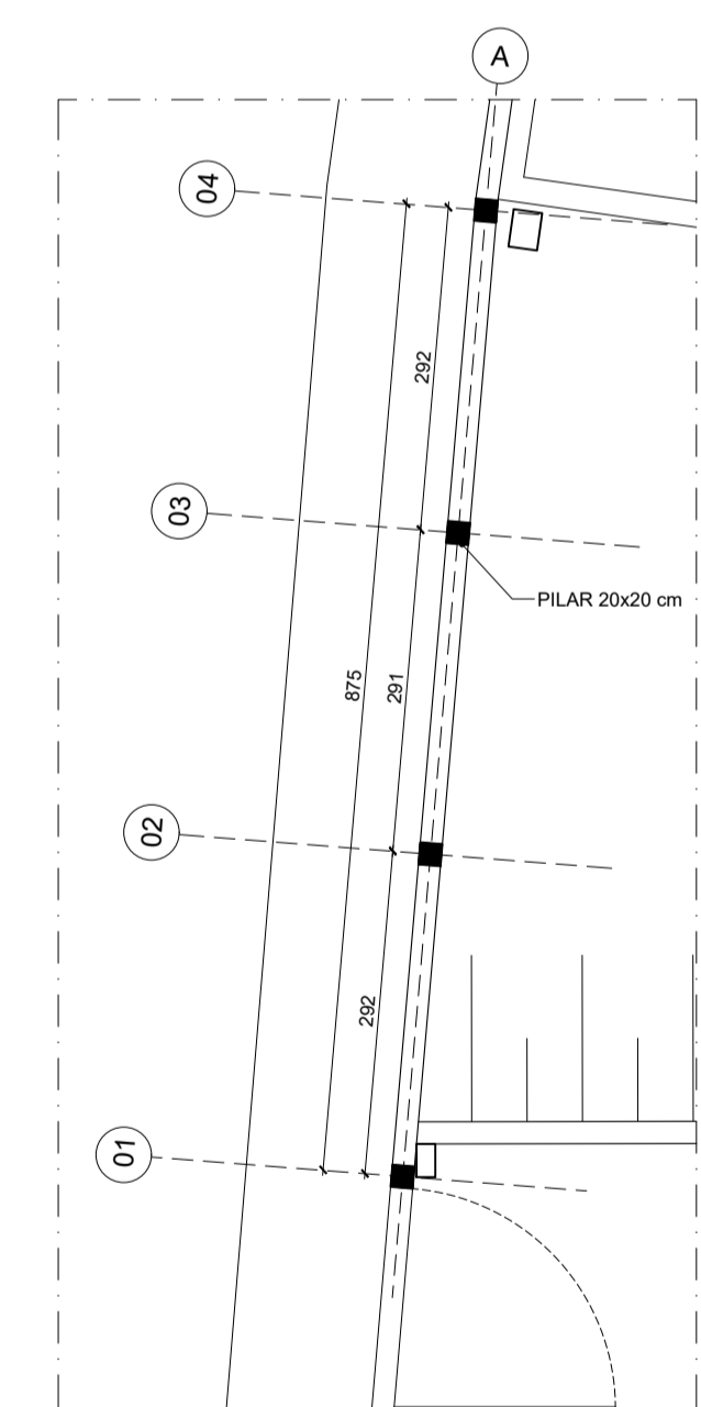
32 PLANTA PILARES - TRECHO 05 ESCALA 1:75
