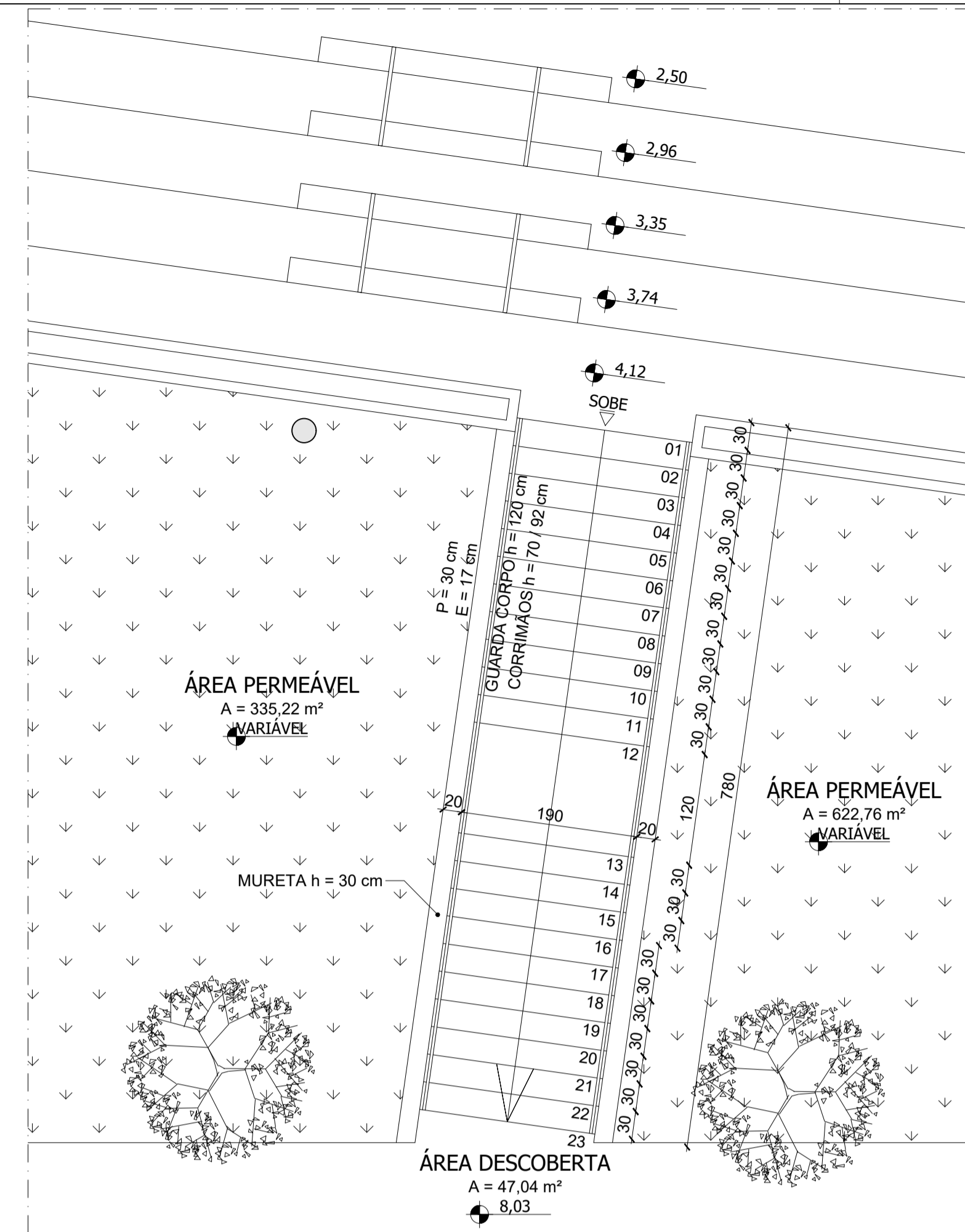
16 PLANTA - ESCADA ESCALA 1:50
