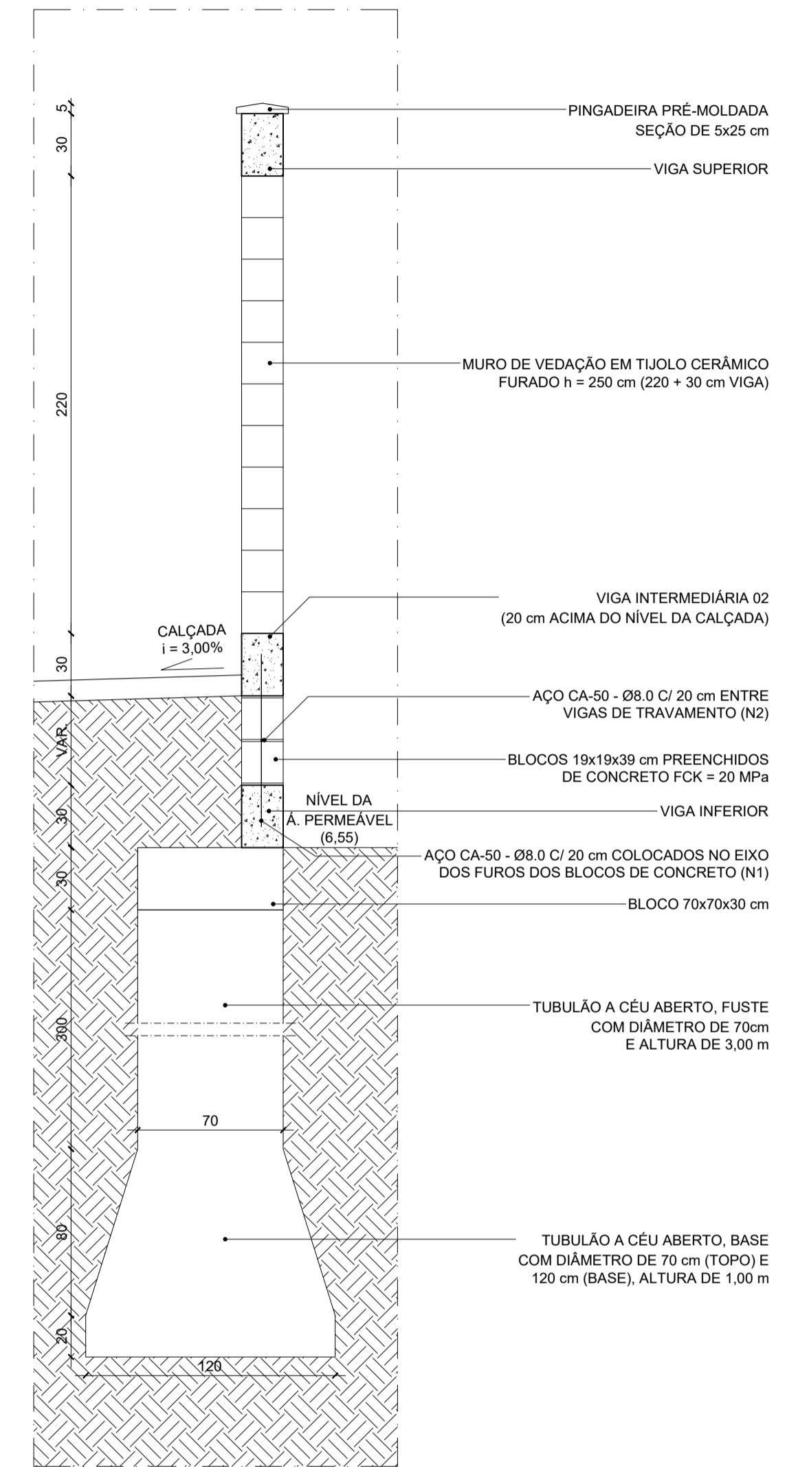
37 SEÇÃO TRANSVERSAL - TRECHO 05 ESCALA 1:25
