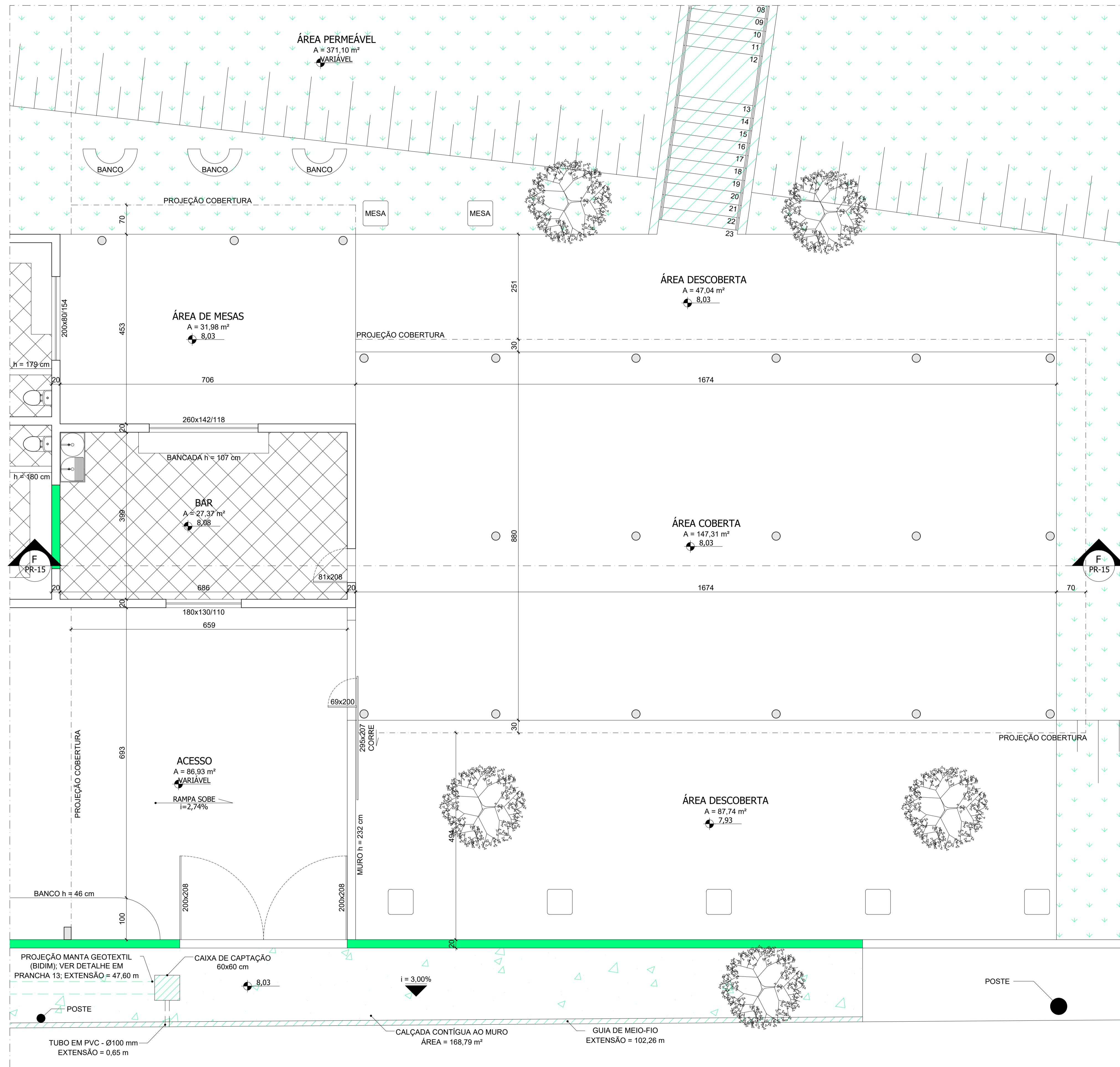
11 PLANTA - BAR (ACRÉSCIMO) ESCALA 1:50
