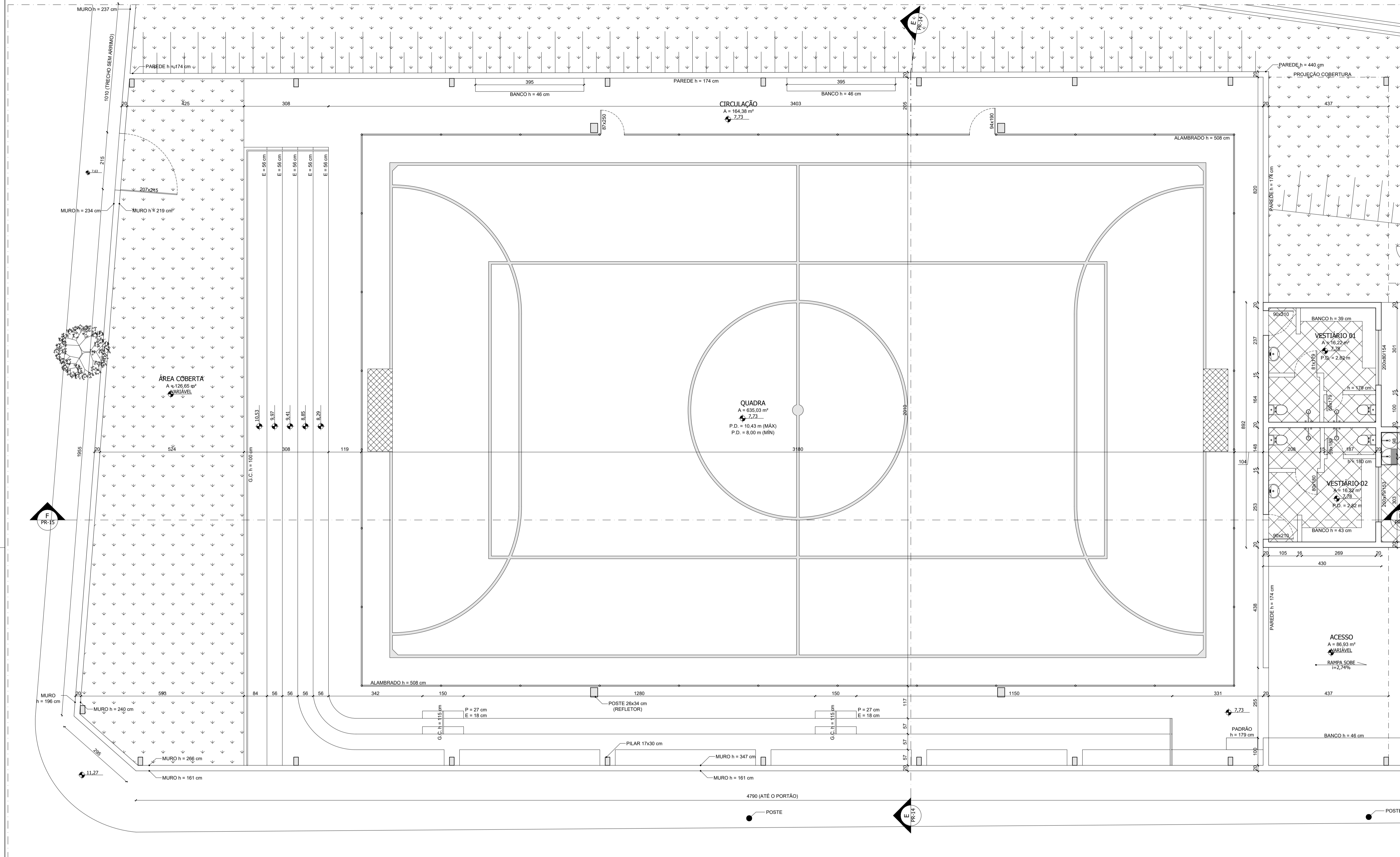
04 PLANTA - QUADRA (EXISTENTE) ESCALA 1:75
