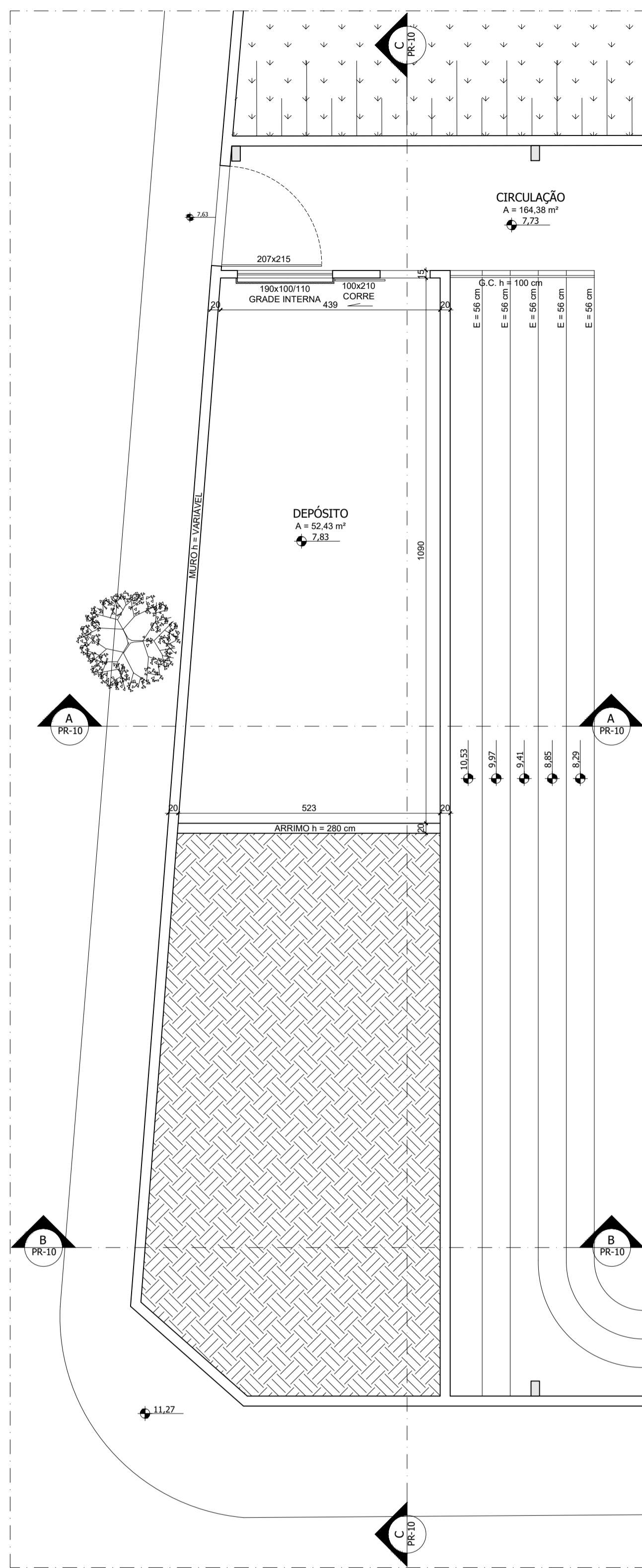
12 PLANTA - DEPÓSITO ESCALA 1:75
