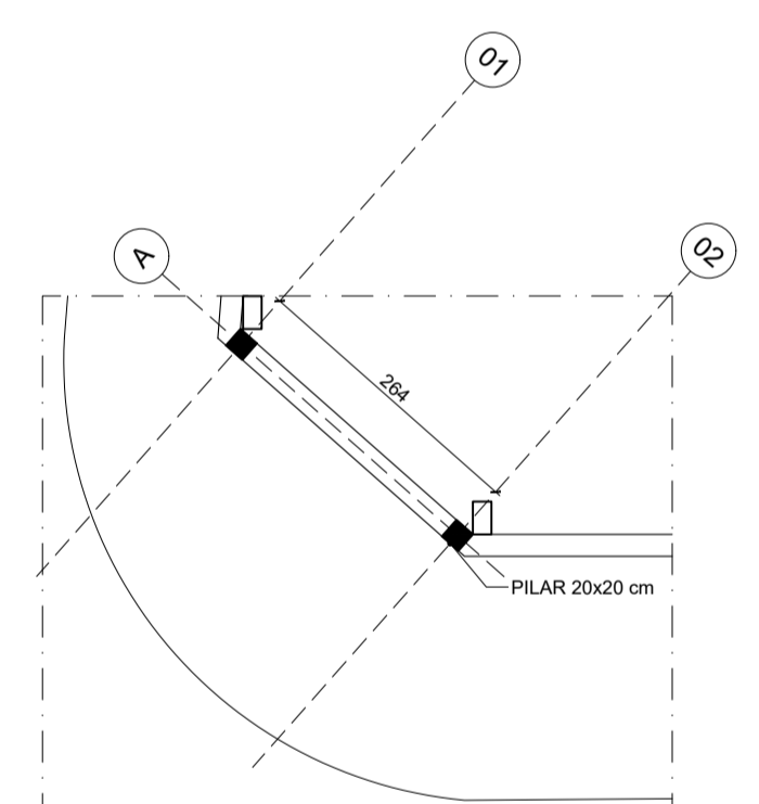
28 PLANTA PILARES - TRECHO 03 ESCALA 1:75
