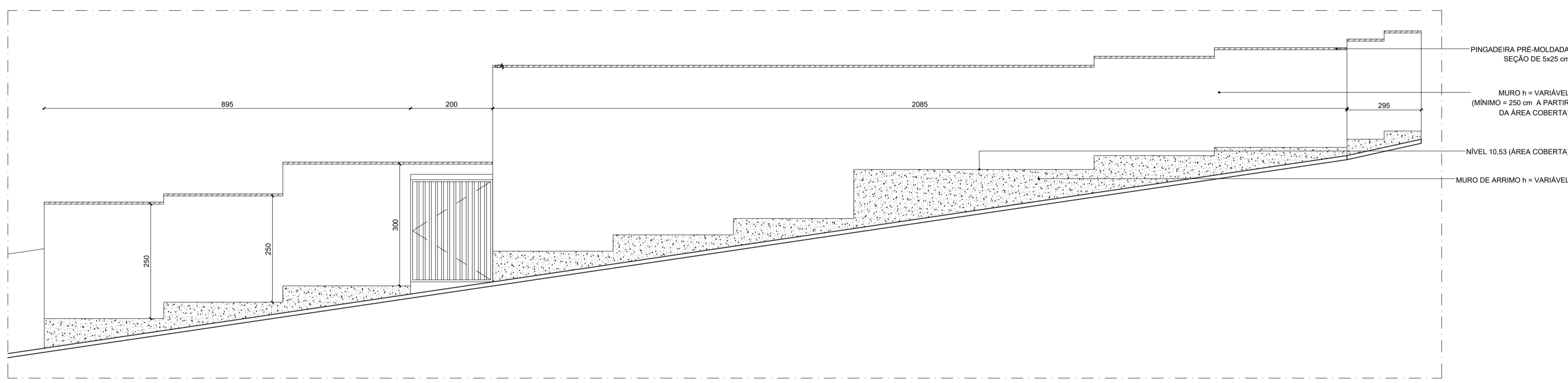
21 ELEVÇÃO 03 ESCALA 1:75
