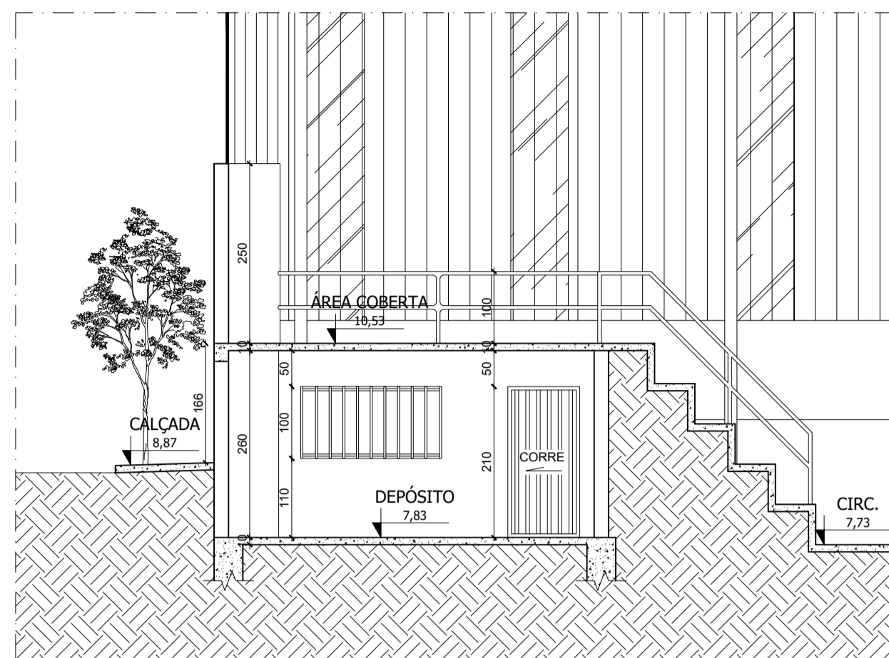
13 CORTE AA ESCALA 1:75
