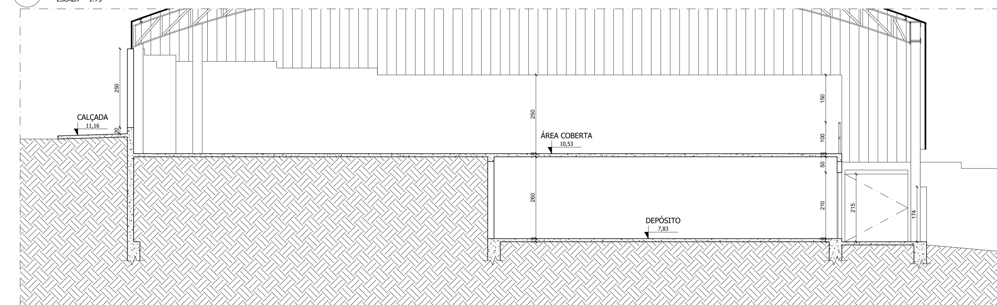
15 CORTE CC ESCALA 1:75
