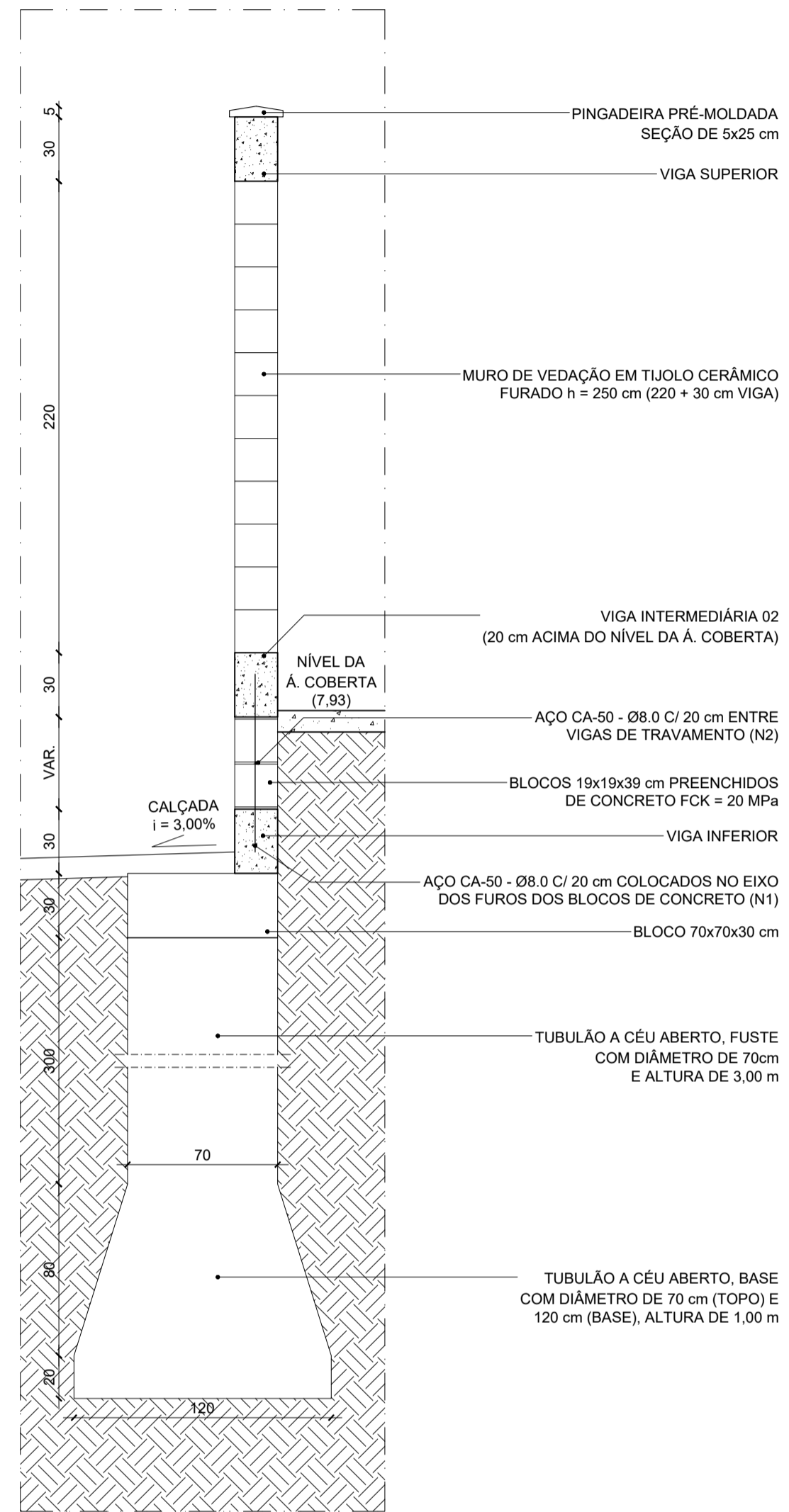
34 SEÇÃO TRANSVERSAL - TRECHO 01 ESCALA 1:25
