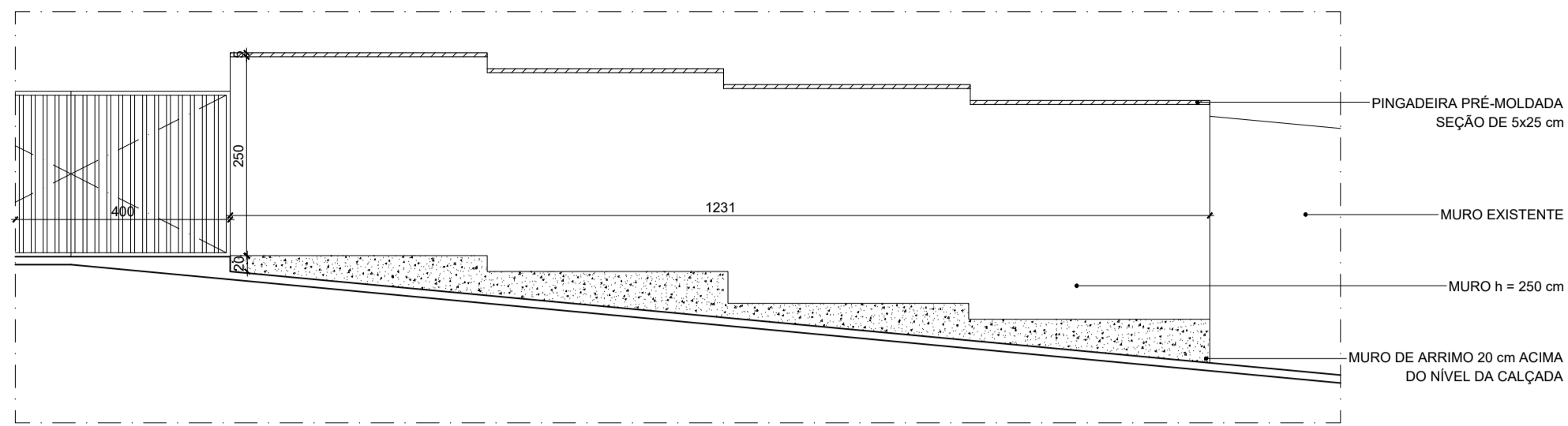
19 ELEVÇÃO 01 ESCALA 1:75
