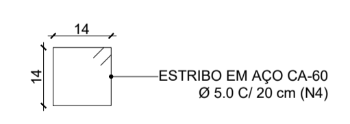
38 DETALHE PILARES ESCALA 1:10
