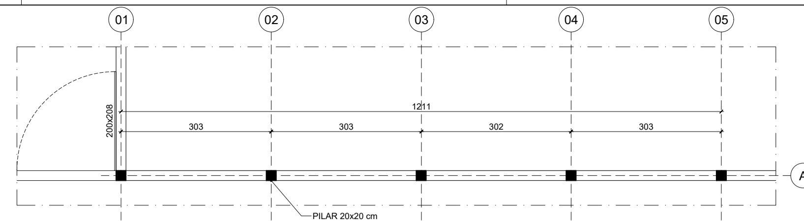
24 PLANTA PILARES - TRECHO 01 ESCALA 1:75
