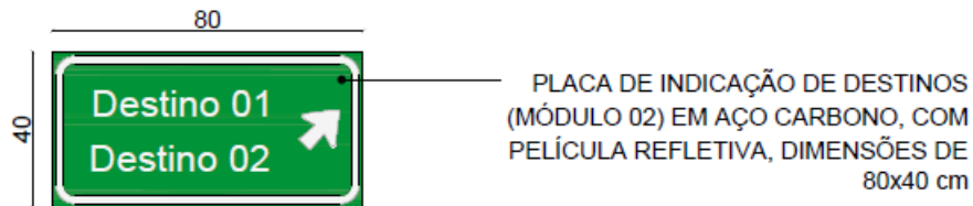
PLACA - SINALIZAÇÃO DE INDICAÇÃO DE DESTINOS SEM ESCALA
