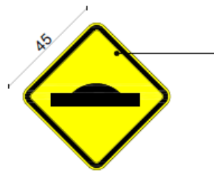
PLACA - SALIÊNCIA OU LOMBADA (A-18) SEM ESCALA
