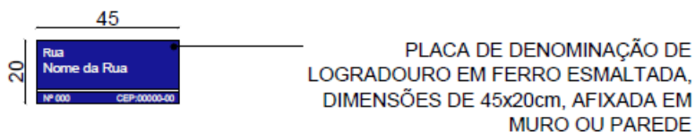
PLACA - DENOMINAÇÃO DE LOGRADOURO SEM ESCALA
