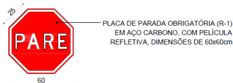
PLACA - PARADA OBRIGATÓRIA (R-1) SEM ESCALA
