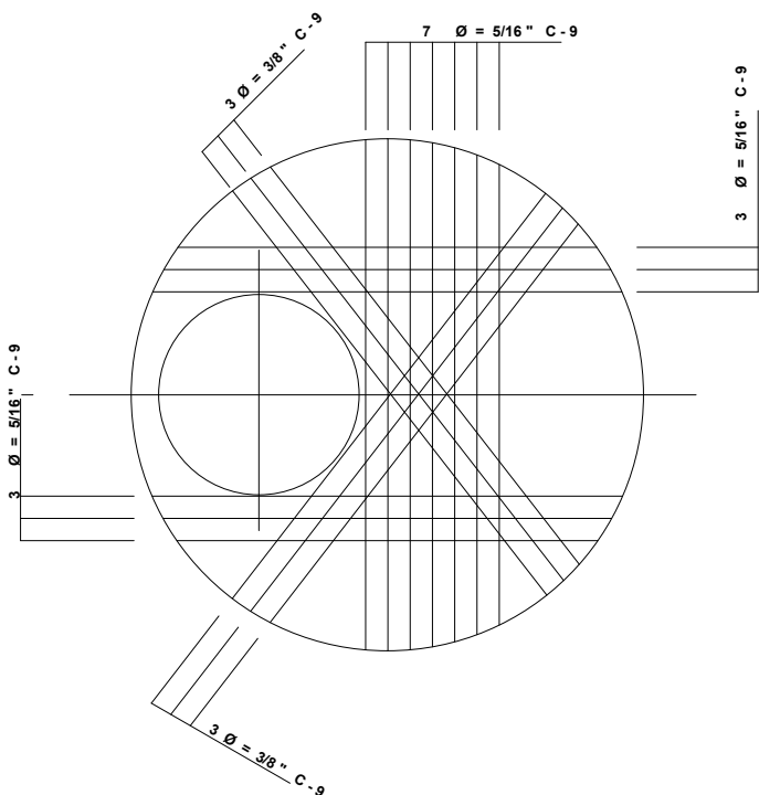
LAJE SUPERIOR DE CONCRETO P.V. DE ESGOTO
