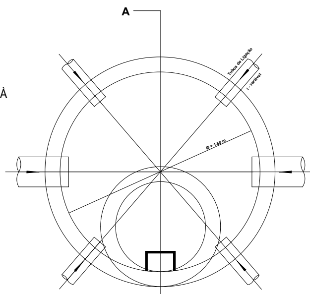
POÇO DE VISITA DE ESGOTO ESC. - 1 : 20
