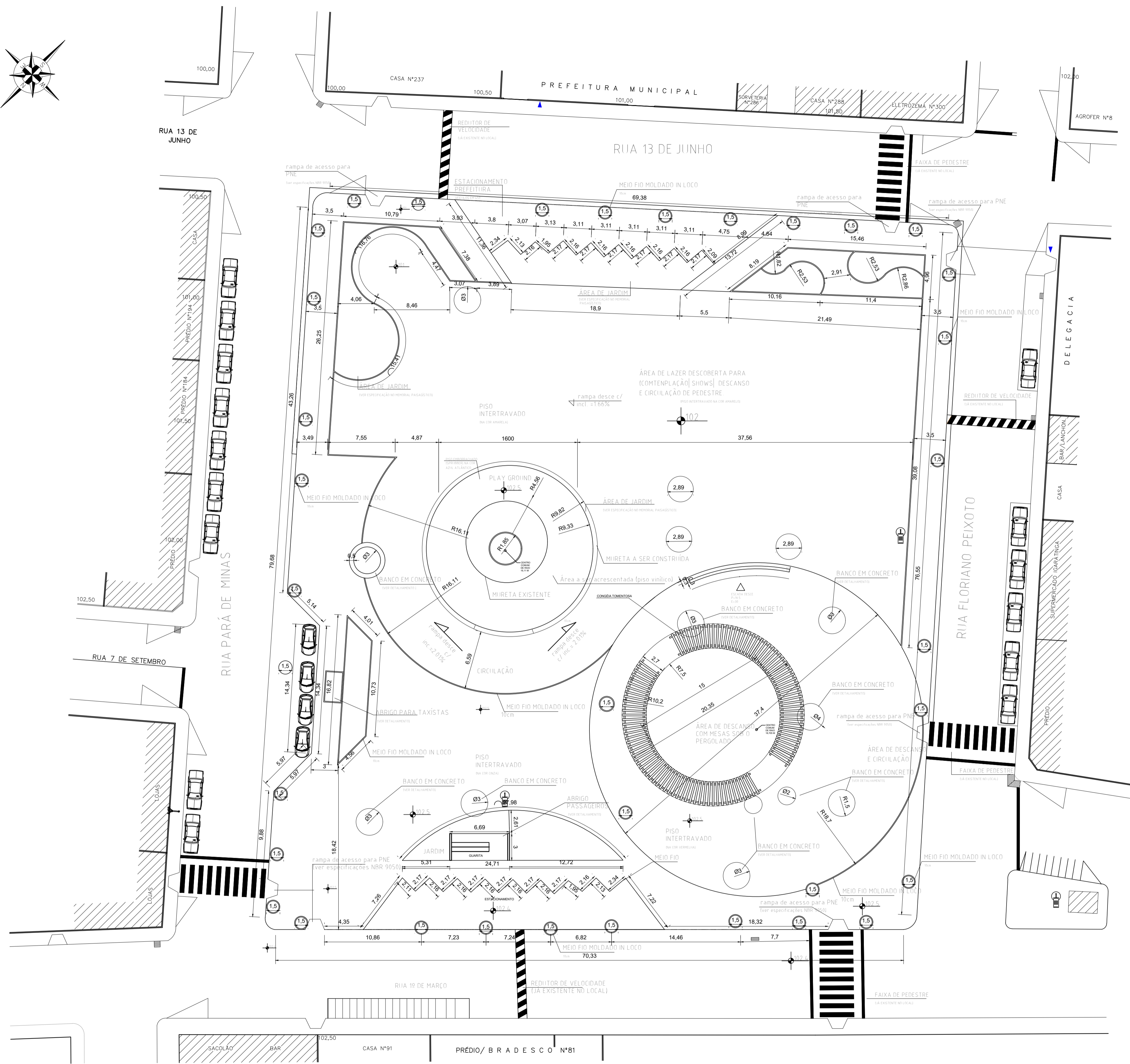
PRAÇA MANOEL DE ASSIS COTAS E ESPECIFICAÇÕES
