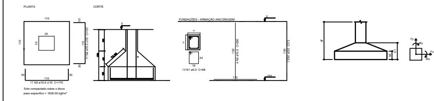
Detalhes dos blocos sem escala
