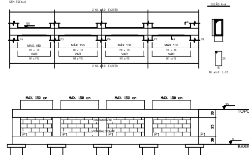
DETALHE DO MURO DE PALCO
