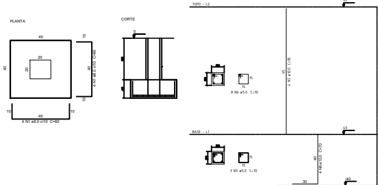
DETALHE TÍPICO DE PILARES PARA PALCO :
