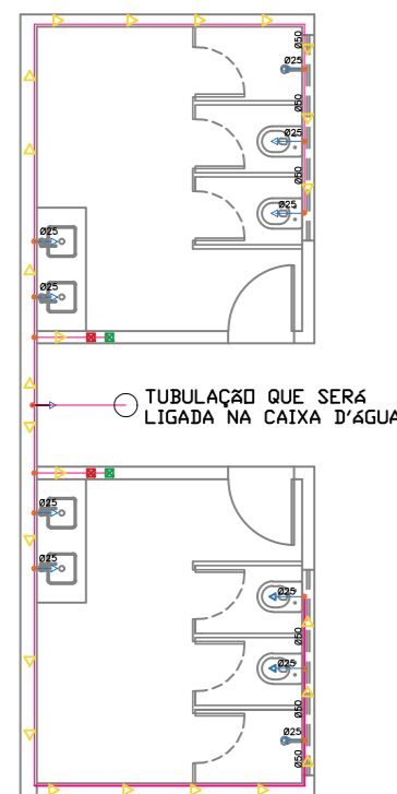
PLANTA BAIXA – ÁGUA FRIA ESCALA 1:100
