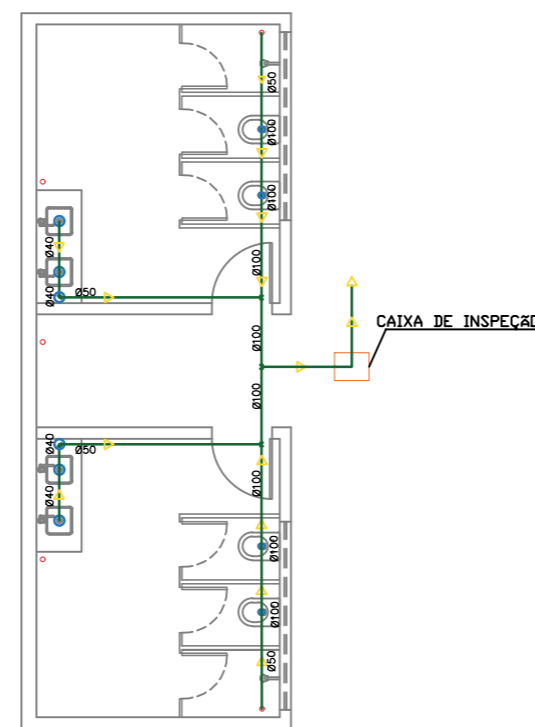
PLANTA BAIXA – ESGOTO ESCALA 1:100
