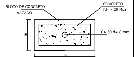
DETALHE B SEM ESCALA
