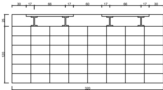
CORTE B-B SEM ESCALA
