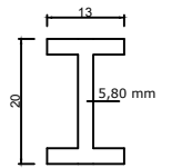
PERFIL W - 200X26,6
